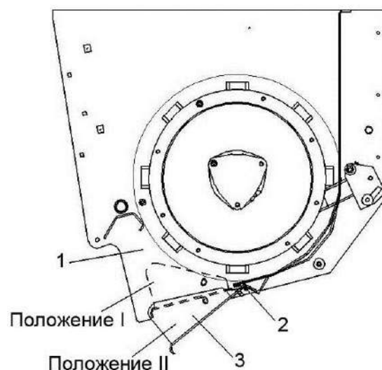
Рисунок 2.19 - Регулировка днища соломоизмельчителя
