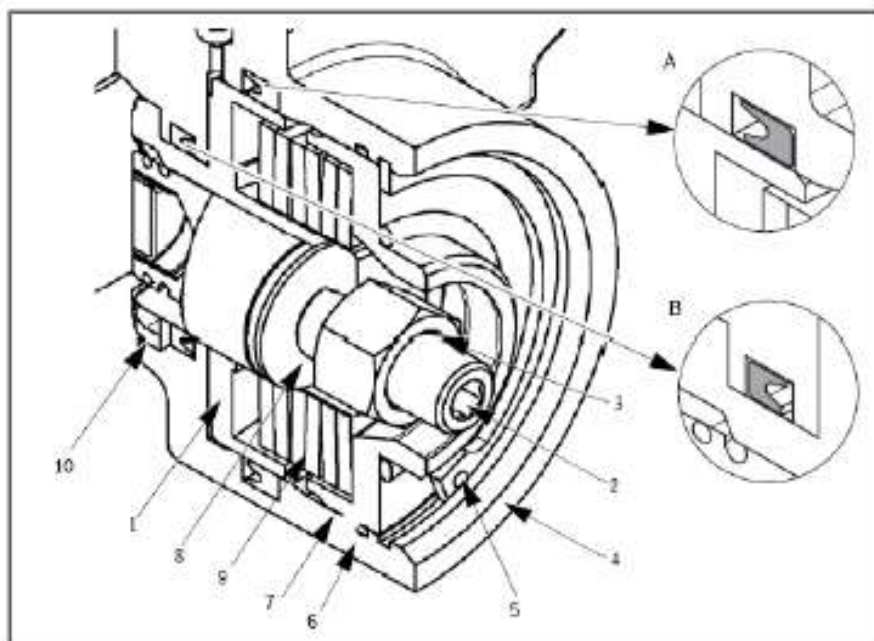
Рисунок 4-3: Замена уплотнений
