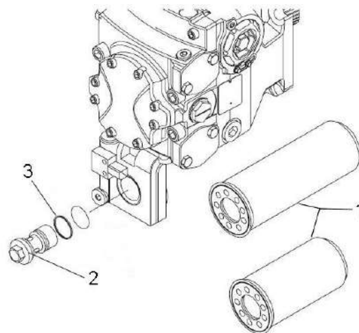
1 – фильтроэлемент; 2 – болт; 3 – уплотнительное кольцо
