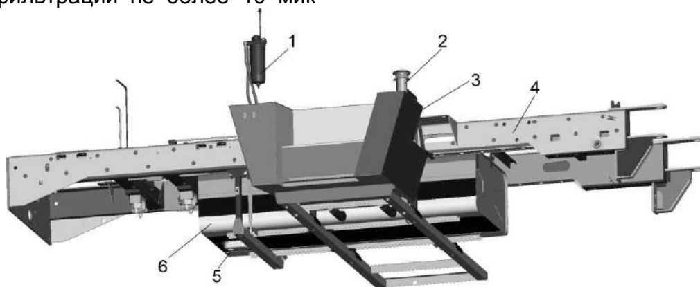
1 – фильтр топливный; 2 – горловина заливная; 3 – бак топливный; 4 – рама; 5 – пробка сливная; 6 – бак топливный
