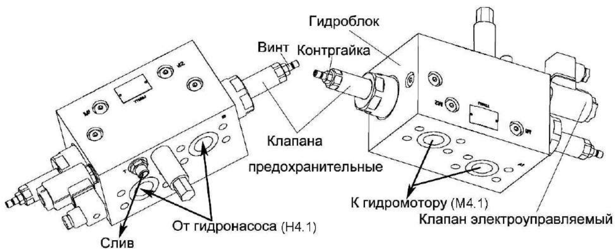
Рисунок 1.61 – Гидроблок адаптеров (ГБ4.1)
