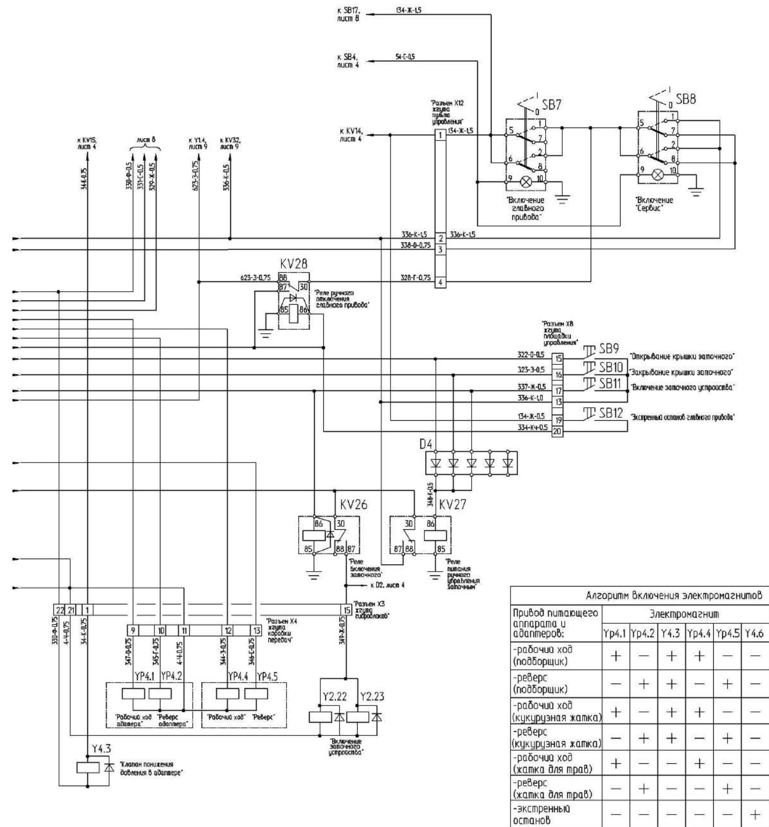
Рисунок В.6 – Схема электрическая принципиальная комплекса (лист 2)
