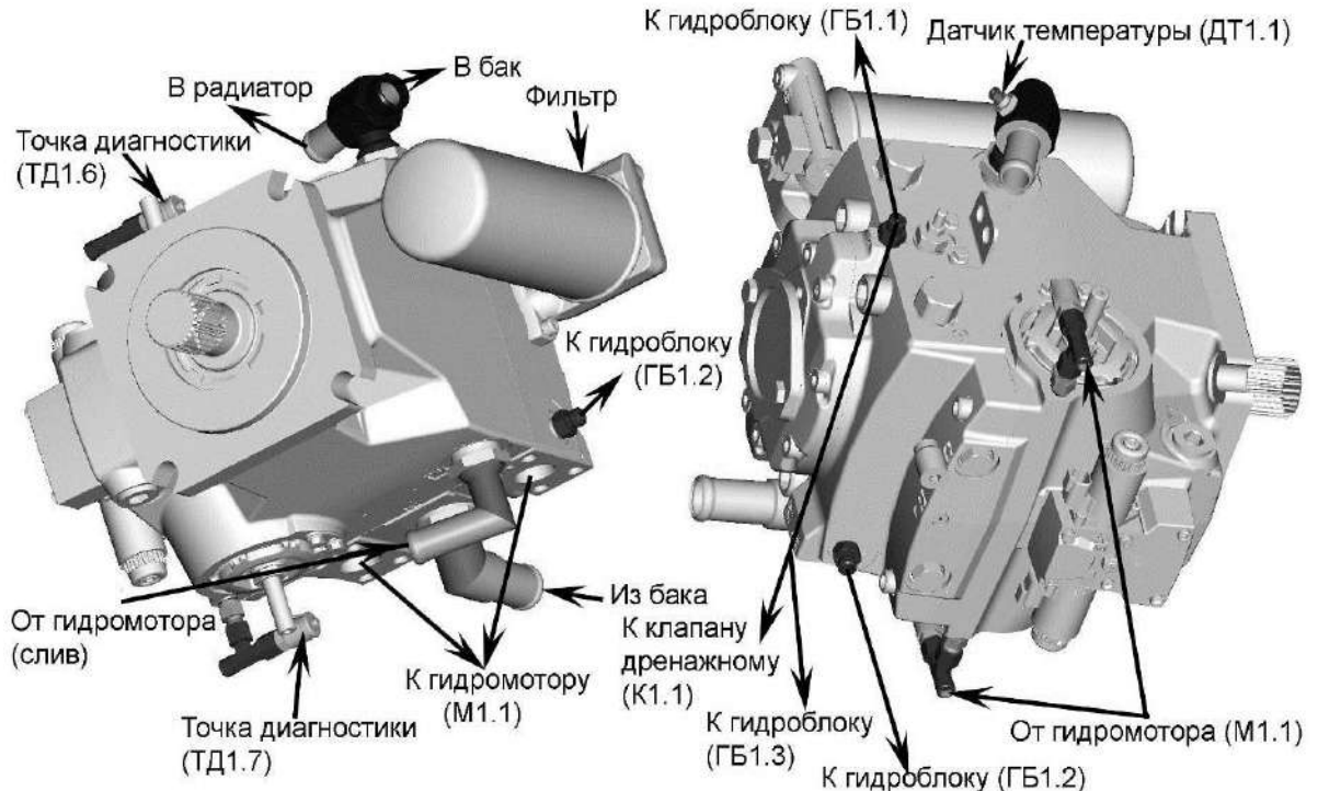
Рисунок 1.35 – Гидронасос привода ходовой части (Н1.1)
