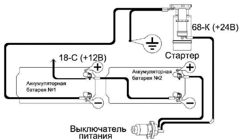
Рисунок 2.1 – Схема подключения аккумуляторных батарей
