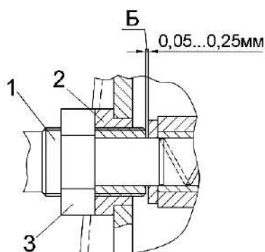
1, 2 – втулки; 3 – гайка
