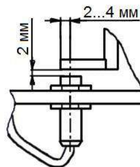
Рисунок 2.14 – Установка датчика положения бруска абразивного
