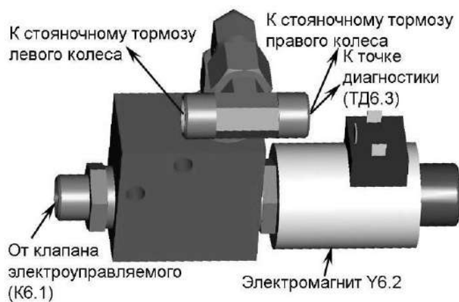
Рисунок 1.69 – Клапан электроуправляемый (K6.2)
