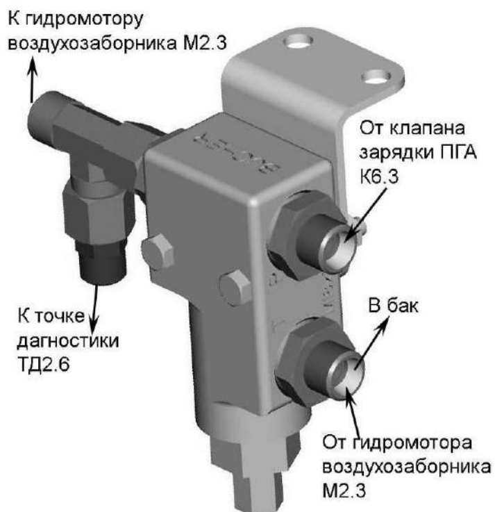
Рисунок 1.53 – Клапан предохранительный (КП2.1)
