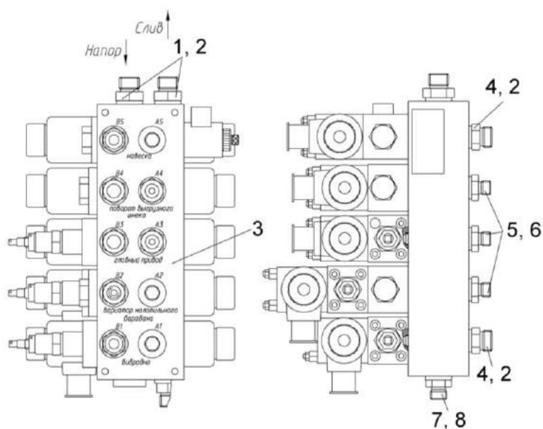
Рисунок 1.20 – Гидроблок пятисекционный
