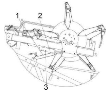
Рисунок 2.37 – Схема установки мотовила
