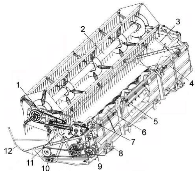
1 – гидроцилиндр выноса мотовила; 2 – мотовило; 3, 11 – гидроцилиндры подъема мотовила по высоте; 4 – рама; 5 – режущий аппарат; 6 – шнек; 7 – вариатор; 8 – копирующий башмак; 9 – исполнительный электромеханизм; 10 – угловая передача; 12 – прутковый делитель
