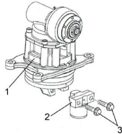
1 – угловая передача; 2 – верхний подпятник; 3 – винт
