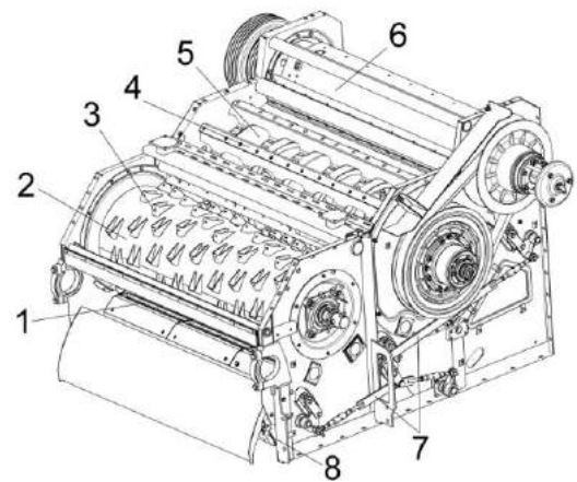
1 – подбарабанье; 2 – барабан ускоряющий; 3 – колпак; 4 – бич; 5 – барабан молотильный; 6 – отбойный битер; 7 – подвески подбарабання; 8 – камнеуловитель
