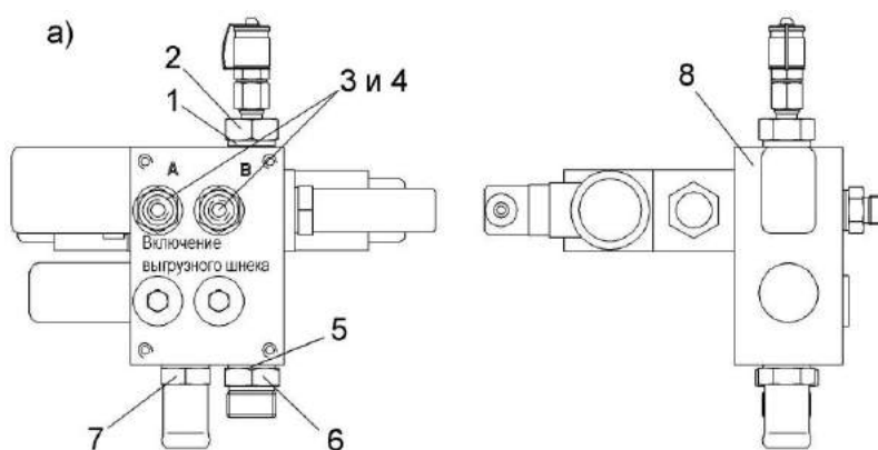
Рисунок 1.22 – Гидроблок односекционный
