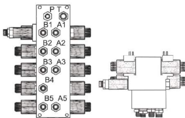
Рисунок 1.21 - Гидроблок пятисекционный
