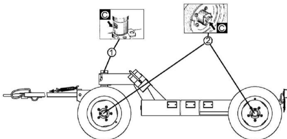
Рисунок 3.4 – Схема смазки транспортной тележки
