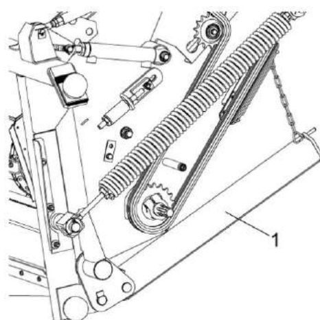
Рисунок 2.13 – Наклонная камера
