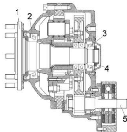
Рисунок 2.27 – Редуктор бортовой
