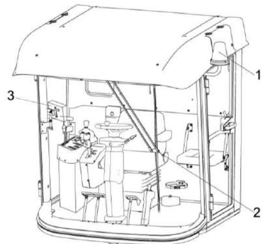
1 – проблесковый маяк; 2 – стеклоочиститель; 3 – модуль терминальный графический
