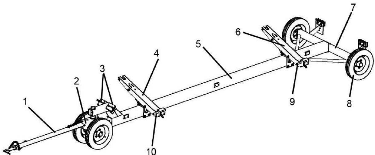
1 –дышло; 2 – ось передняя; 3 - упоры; 4, 6 – ложементы; 5 - рама; 7 –балка габаритная; 8 – колесо; 9, 10 – фиксаторы
