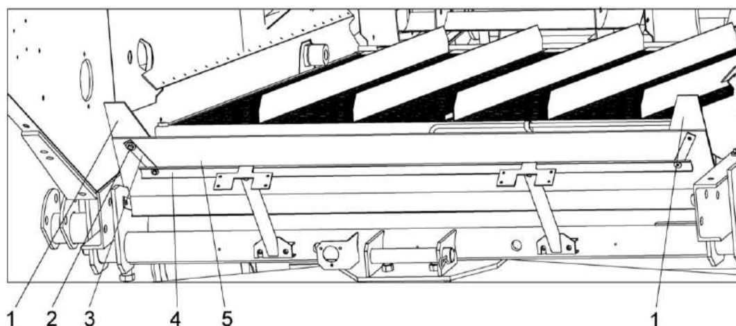
1 - дополнительные щитки; 2 - детали крепления; 3, 4 - планки; 5 - щиток
