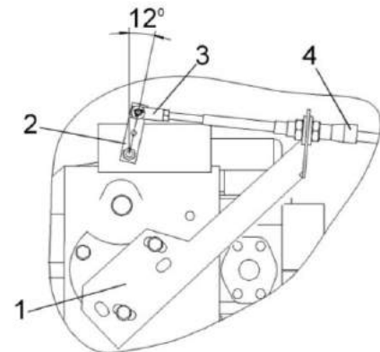
1 – кронштейн; 2 – флажок гидронасоса; 3 – ось; 4 – трос
