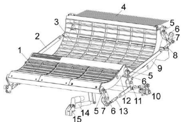
1 – деки переднего подбарабання; 2, 8, 10, 13 – тяги; 3 – дека заднего подбарабання; 4 – решетка пальцевая; 5 – фиксаторы; 6 – стяжки; 7, 11 – рычаги; 9 – каркас заднего подбарабання; 12 – каркас переднего подбарабання; 14 – электромеханизм; 15 – кронштейн
