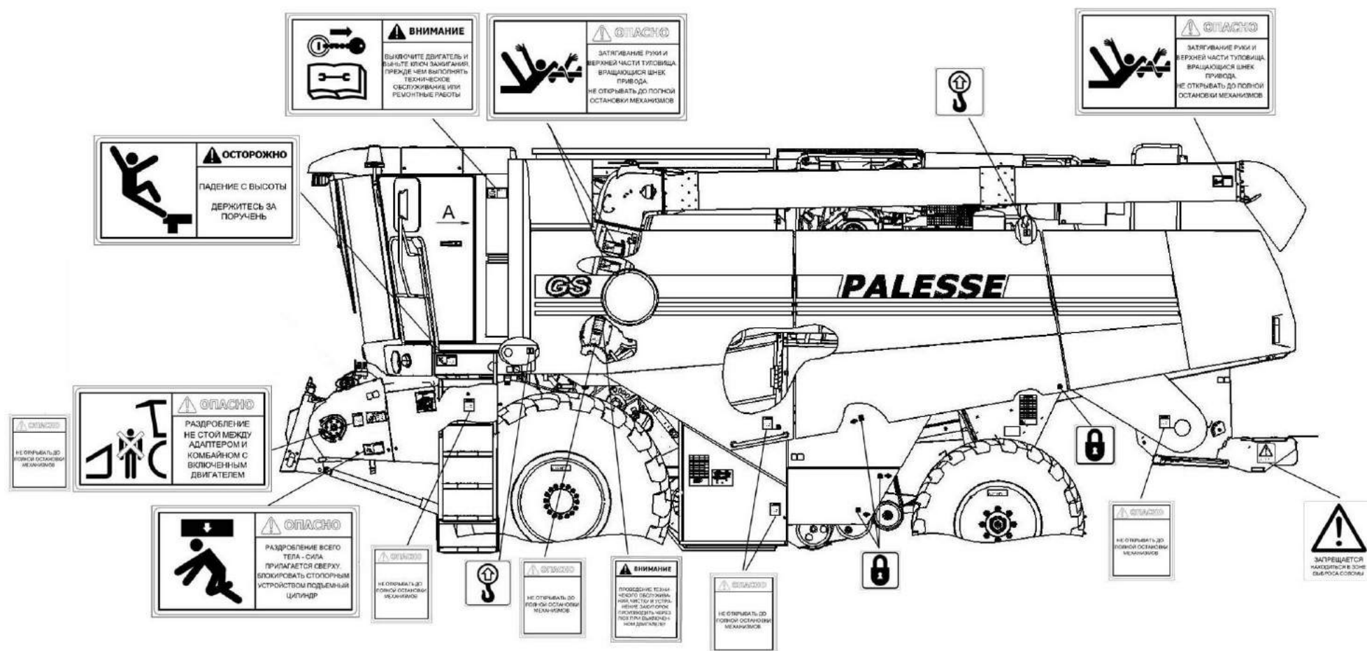
Молотилка самоходная (вид слева)
