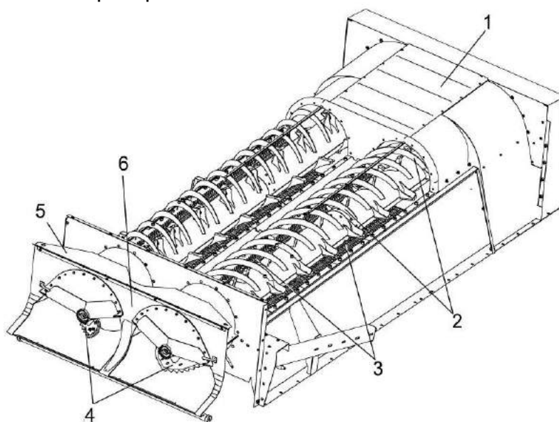
Рисунок 1.12 – Соломосепаратор
