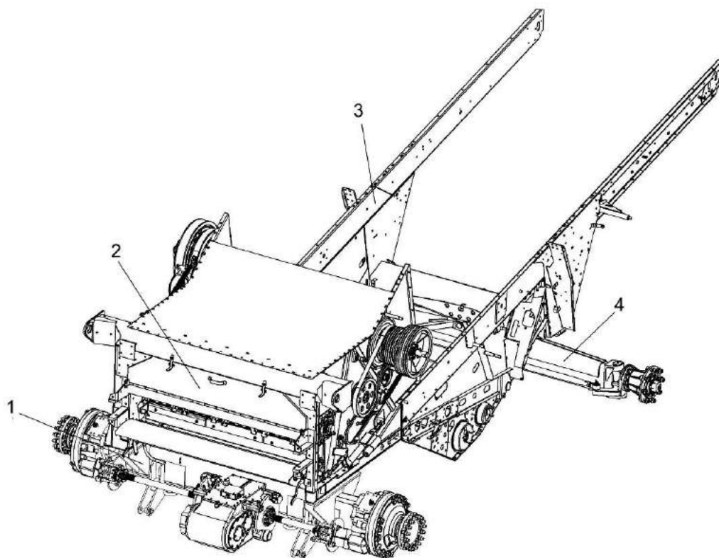
Рисунок 1.6 – Шасси
