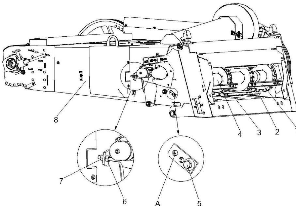
Рисунок 2.15 – Камера наклонная
