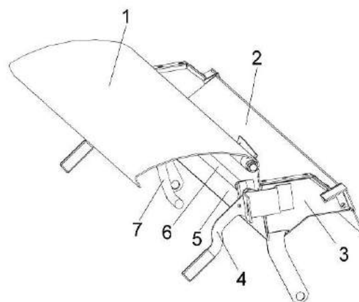
Рисунок 1.9– Аппарат молотильный
