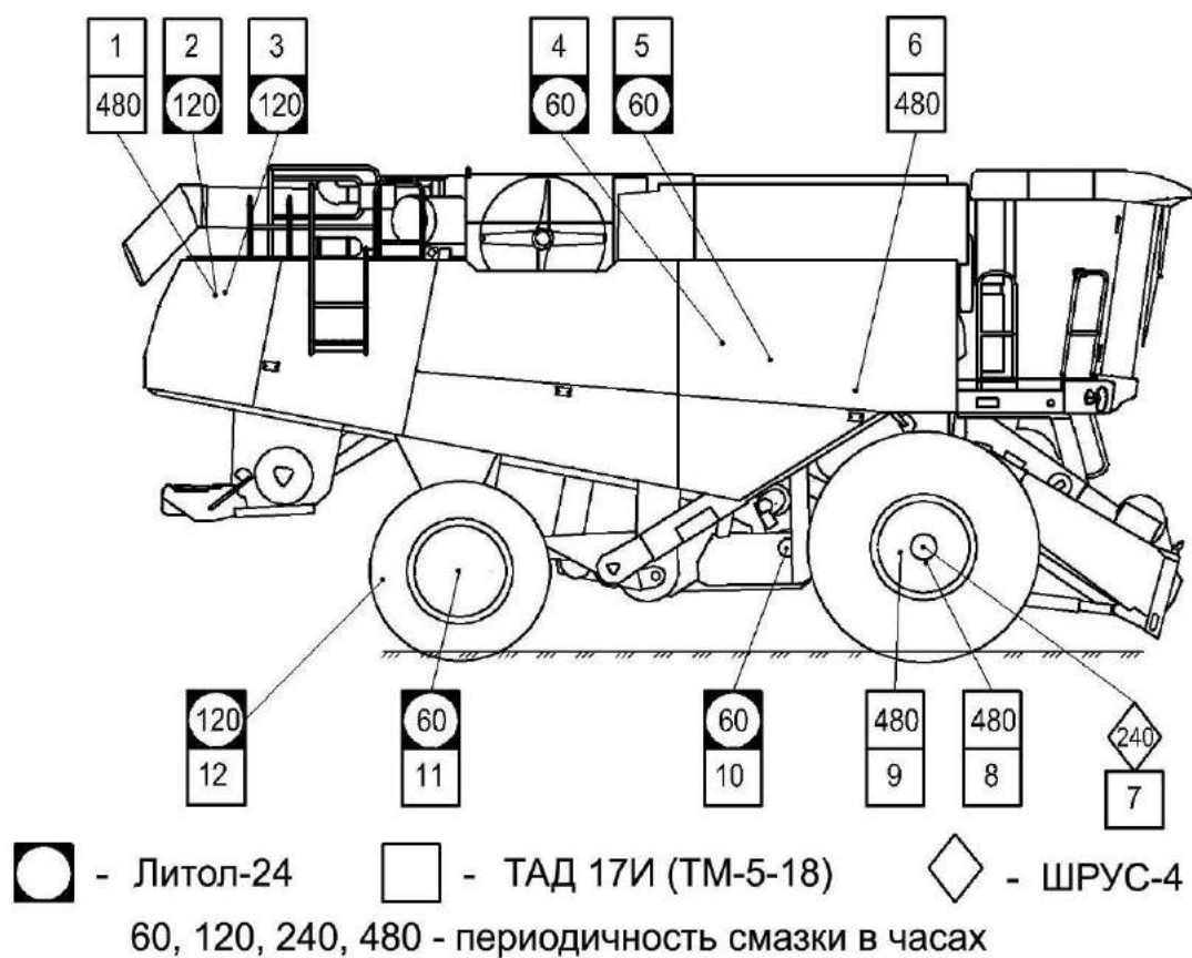
Рисунок 3.1 – Смазка молотилки самоходной (вид справа)
