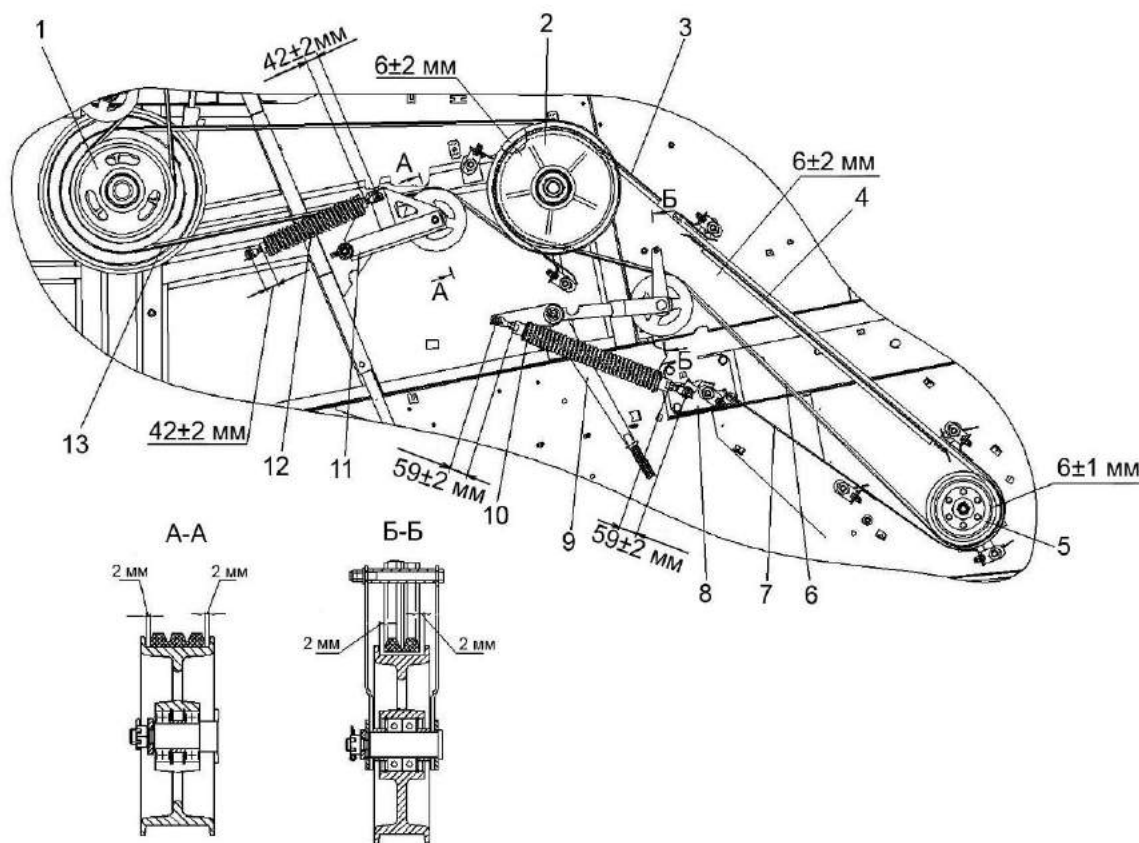
Рисунок 2.8 - Привод соломоизмельчителя
