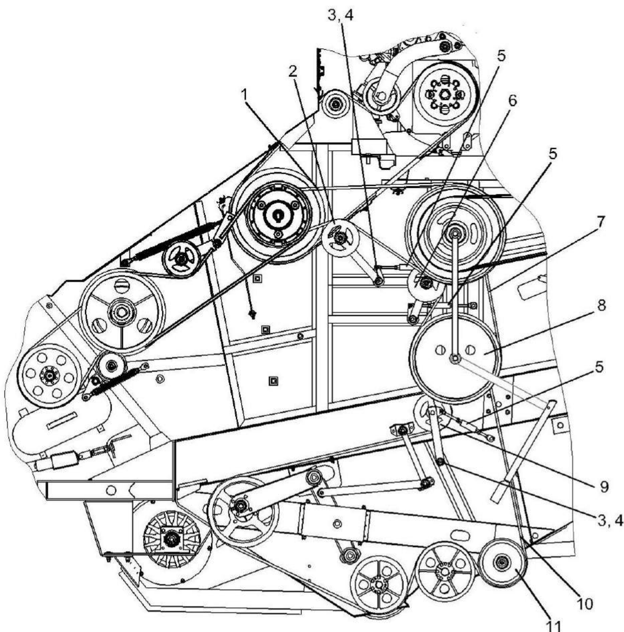
Рисунок 2.6а – Регулировка привода очистки
