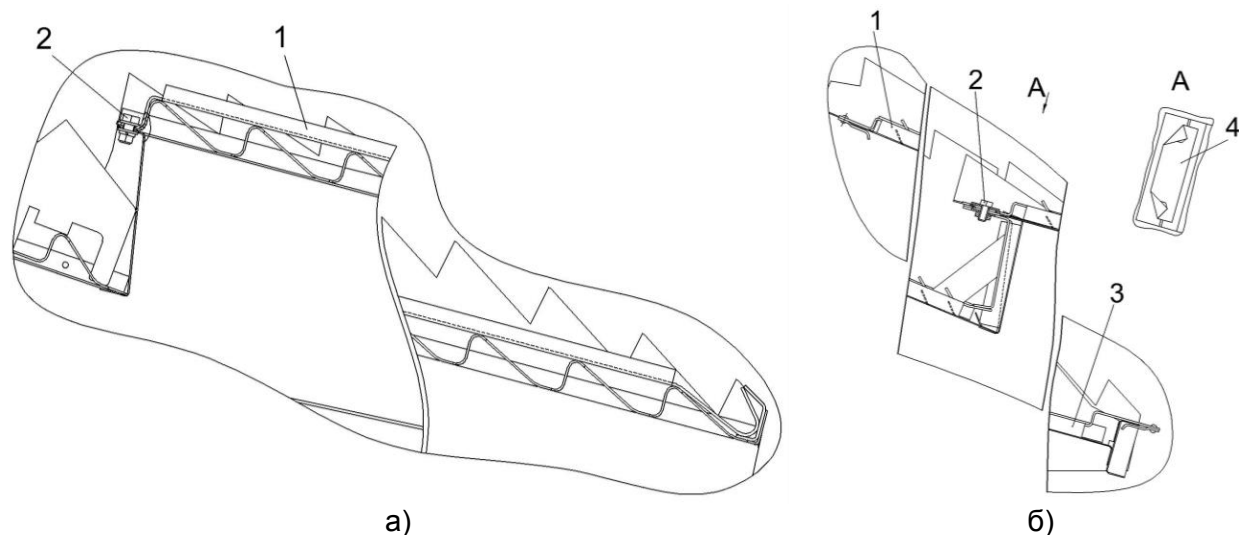
1, 3 – щиток, 2 – болт; 4 – пластина
