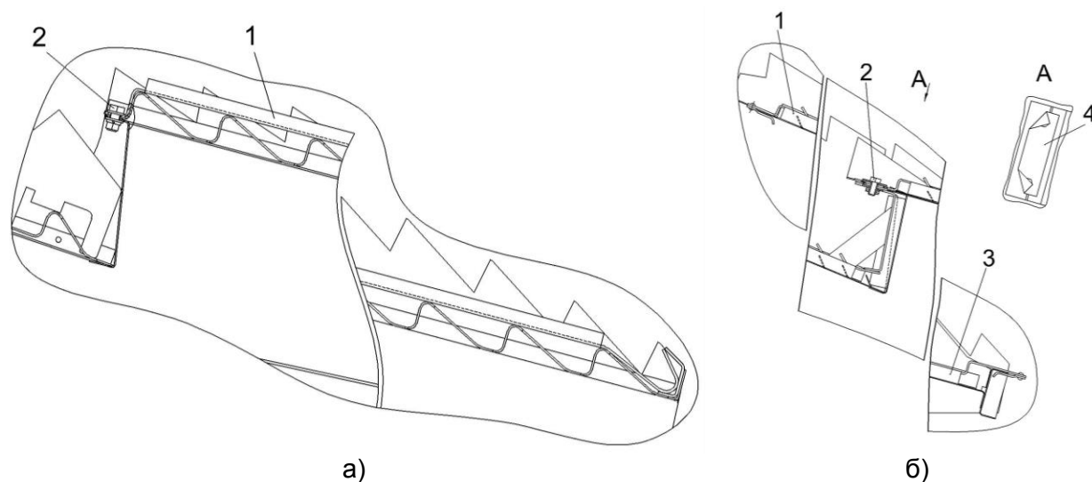
1, 3 - щиток, 2 – болт; 4- пластина
