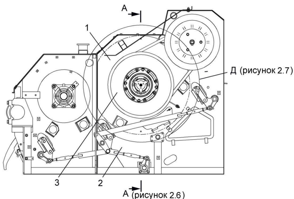
1 – фланец; 2 – аппарат молотильный; 3 – вариатор барабана
