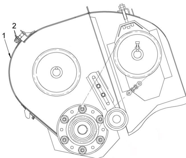
1 – крышка; 2 – гайки
