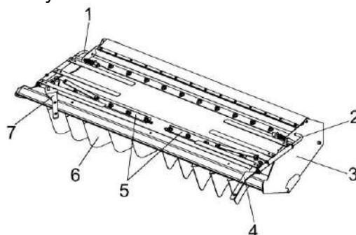
Рисунок 2.11 – Соломоизмельчитель
