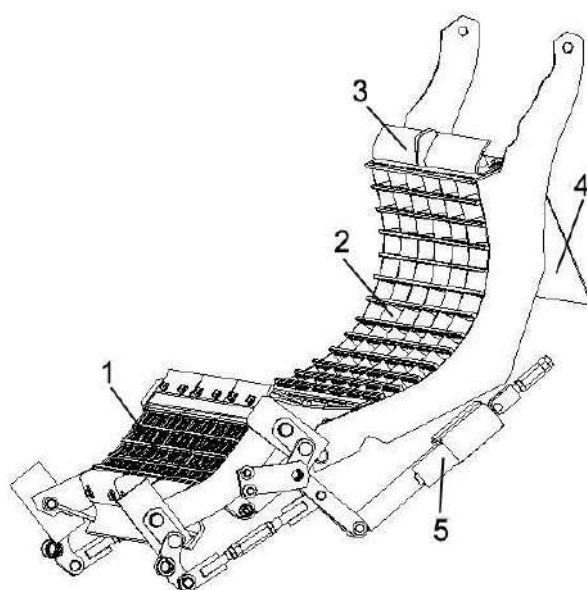
Рисунок 1.10 – Камнеуловитель
