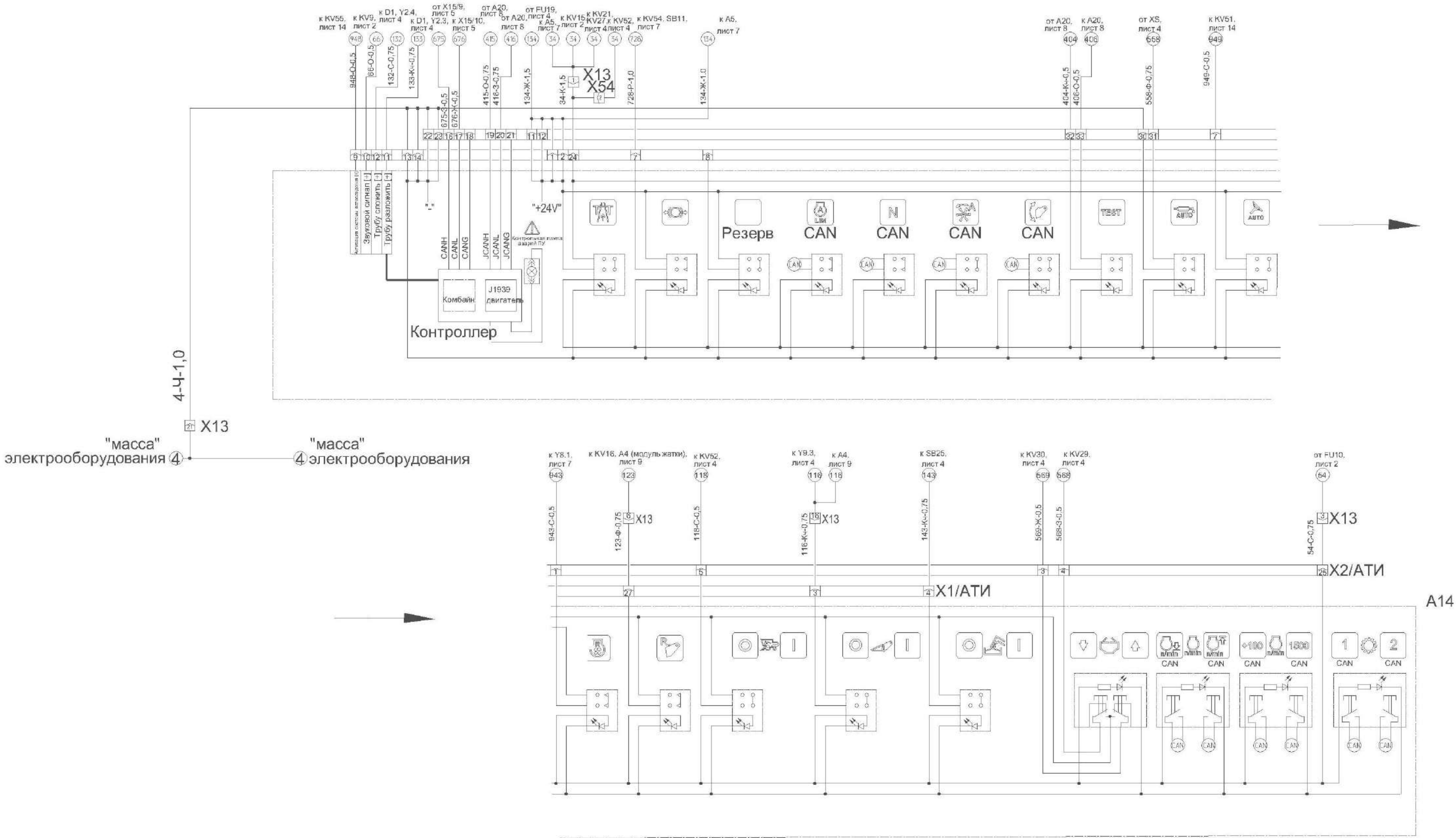
Рисунок Б.15 – Схема электрическая принципиальная комбайна (лист 15)
