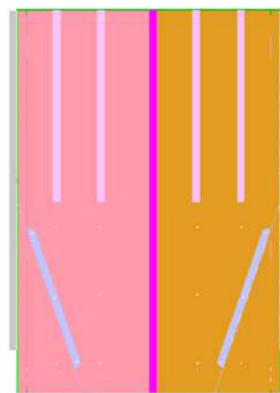
Рисунок 2.15 - Скатная доска. Положение делителей при забивании массы по краям доски
