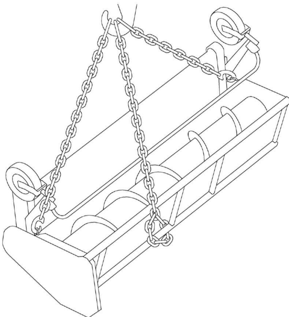
Рисунок 6.1 – Схема строповки
