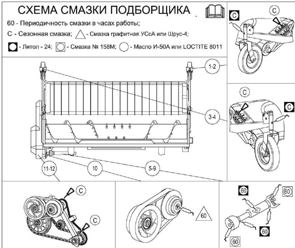
Рисунок 3.1 – Схема смазки
