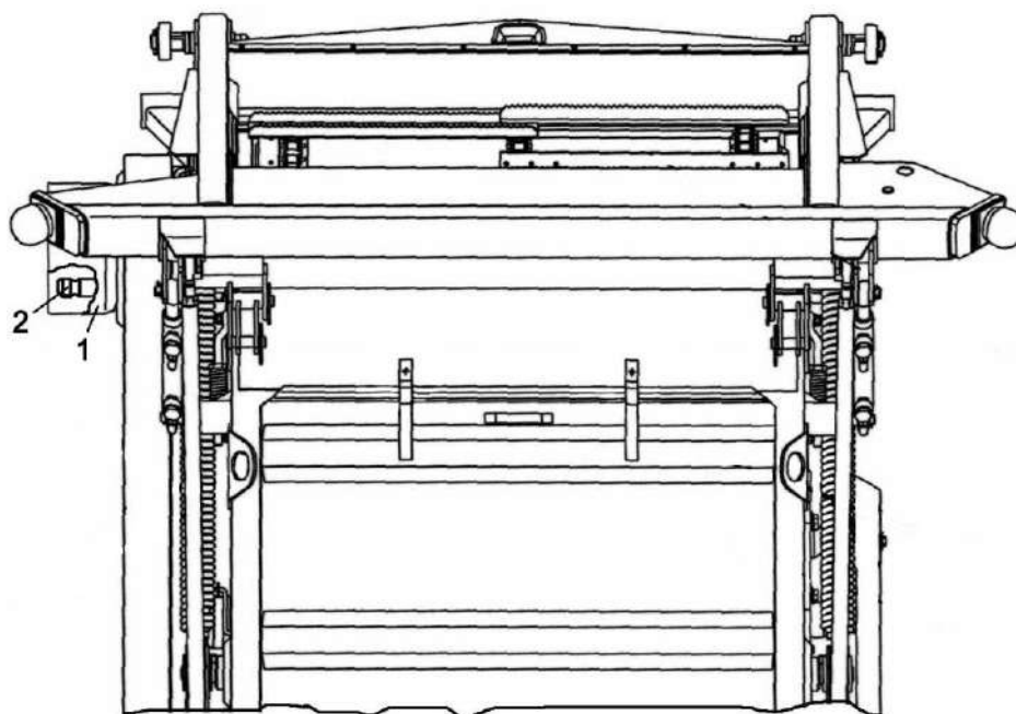
Рисунок 2.2 – Установка карданного вала на вал наклонной камеры
