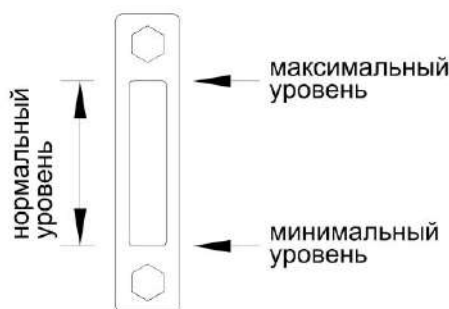
Рисунок 2.6 – Маслоуказатель
