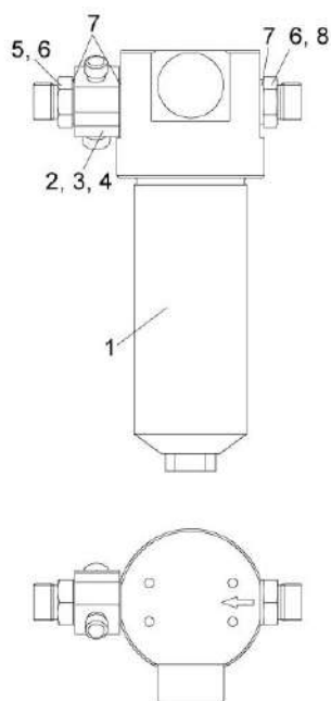
Рисунок 1.23 – Фильтр сливной
