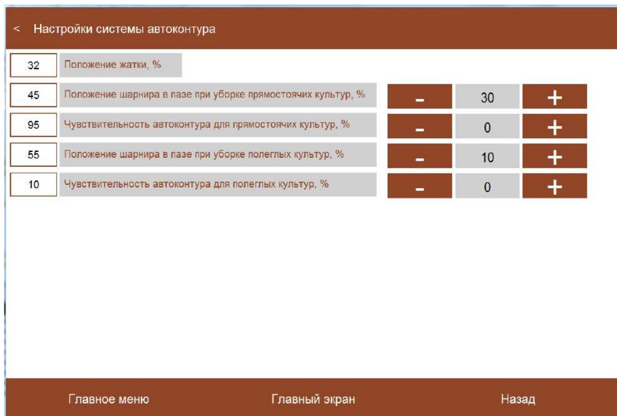
Рисунок А.7 – Экран «Настройки системы автоконтура»
