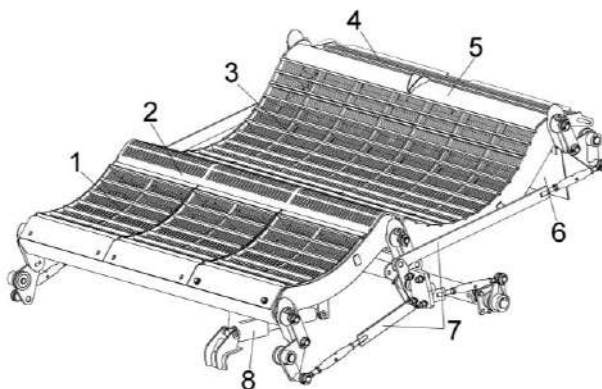
1 – переднее подбарабанье; 2 – решетка; 3 – заднее подбарабанье; 4 – решетка; 5 – козырек; 6 – фартук; 7 – механизм подъема подбарабаний; 8 – электромеханизм
