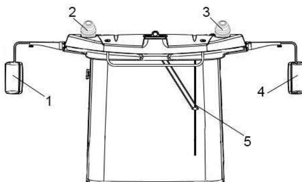
1, 4 – зеркала; 2, 3 – маяк проблесковый; 5 – стеклоочиститель
