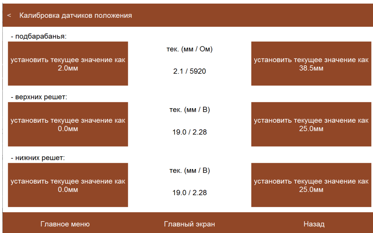
Рисунок А.6 – Экран «Калибровка датчиков положения»
