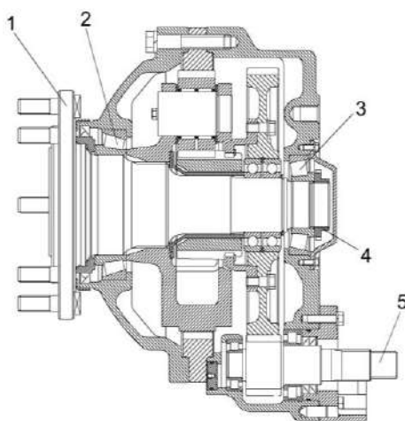
1 – колесо; 2, 3 – подшипники; 4 – гайка; 5 – вал-шестерня
