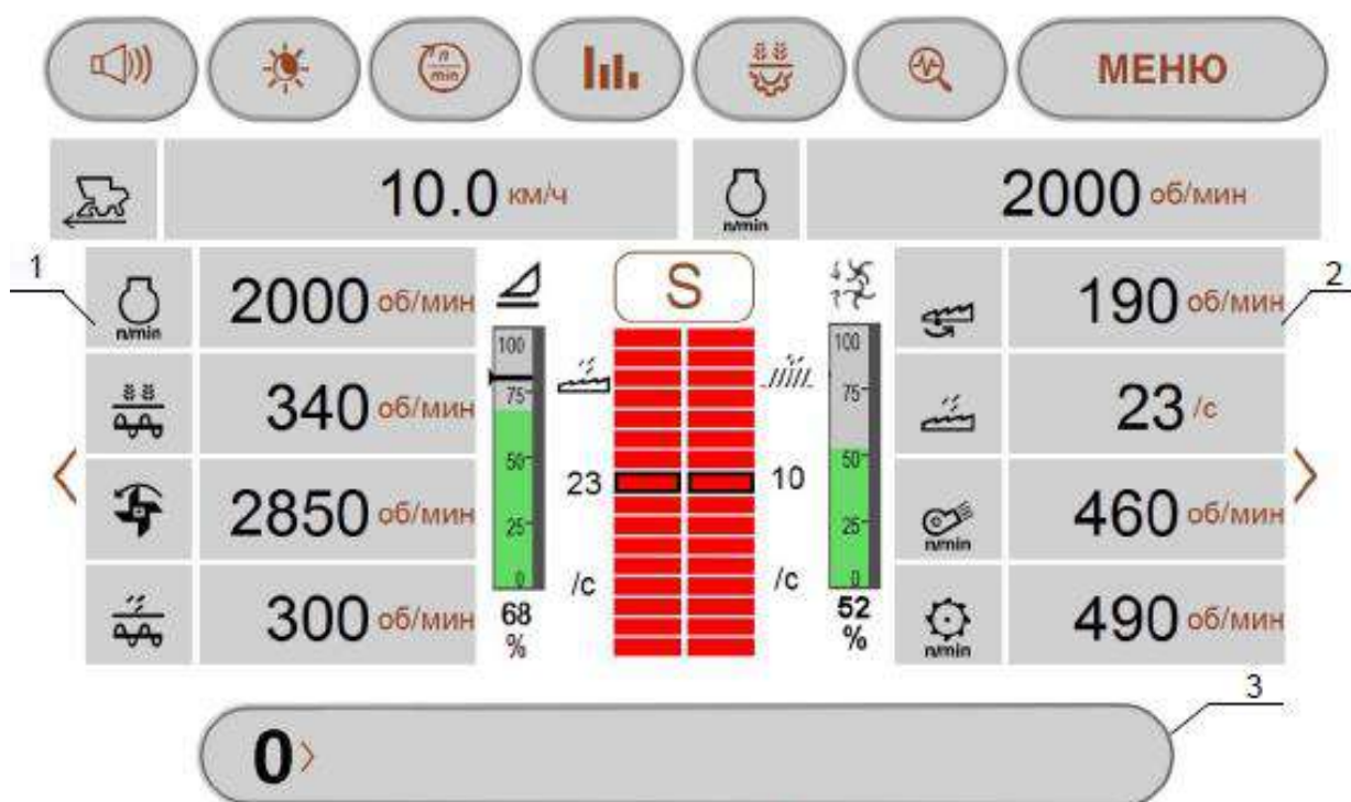
Рисунок А.2 – Экран «КОМБАЙНИРОВАНИЕ»
