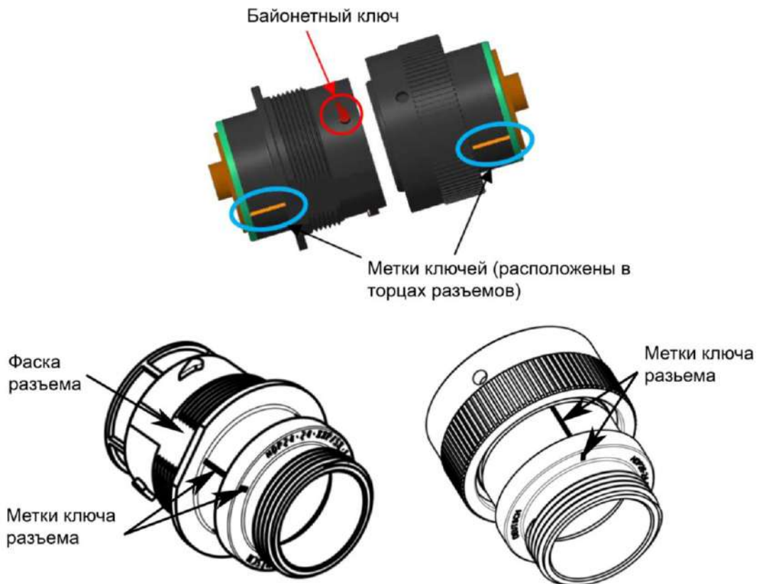
Рисунок 2.13 – Совмещение по ключам
