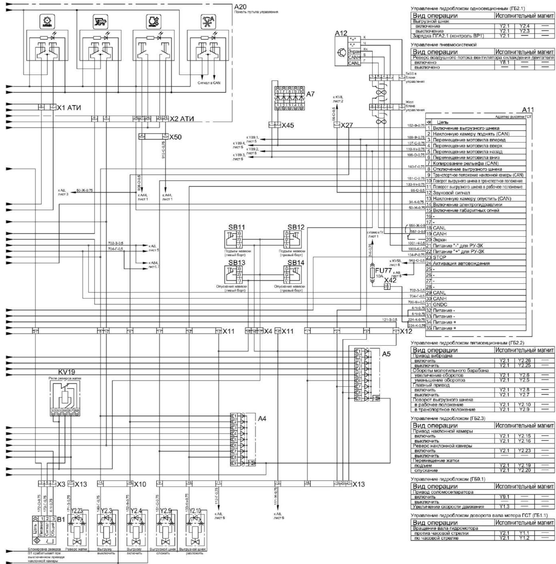
Рисунок Б.4 – Схема электрическая принципиальная комбайна (лист 4)
