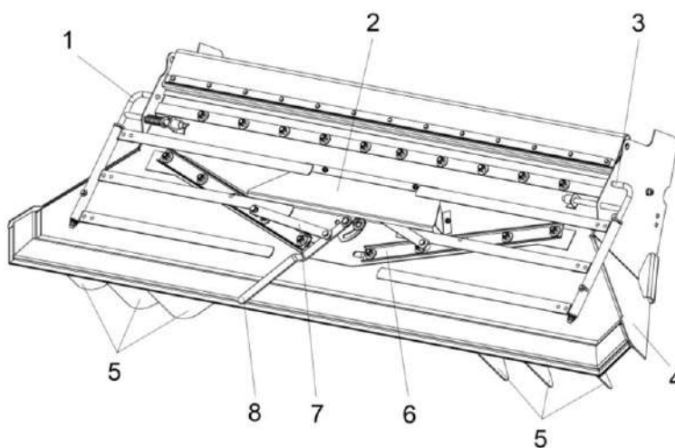
1, 3 – граблины; 2 – крышка; 4 – кожух; 5 – лопатки; 6 – планка регулировочная; 7 – планка; 8 – рукоятка сектора
