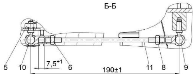
Расположение датчика В13
