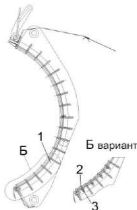
1 – подбарабанье; 2 – планка; 3 – гайка
