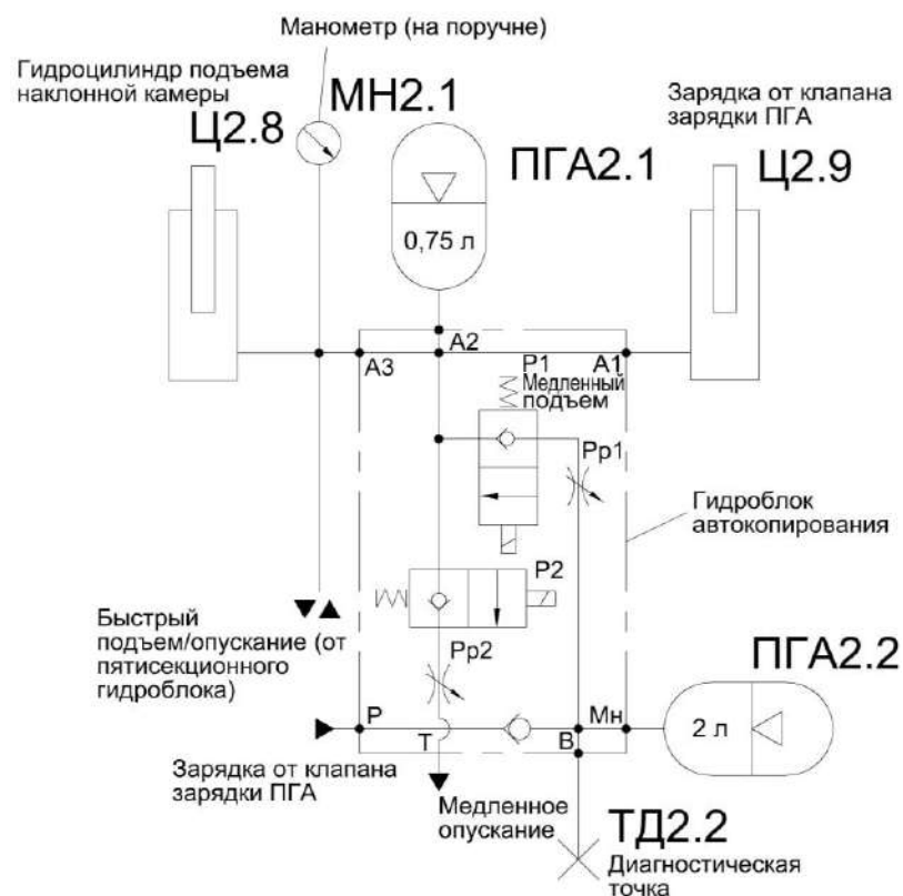
Рисунок 1.21 – Схема гидравлическая гидроблока автокопирования
