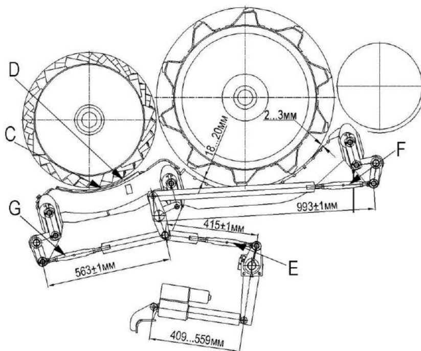
Рисунок 2.18 – Схема молотильного аппарата
