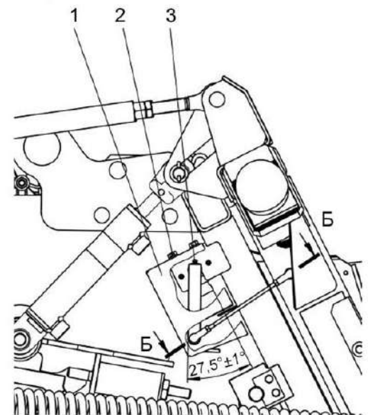
Расположение датчика В13
