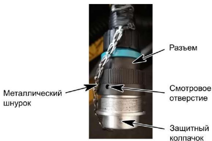
Рисунок 2.17 – Соединение защитного колпачка
