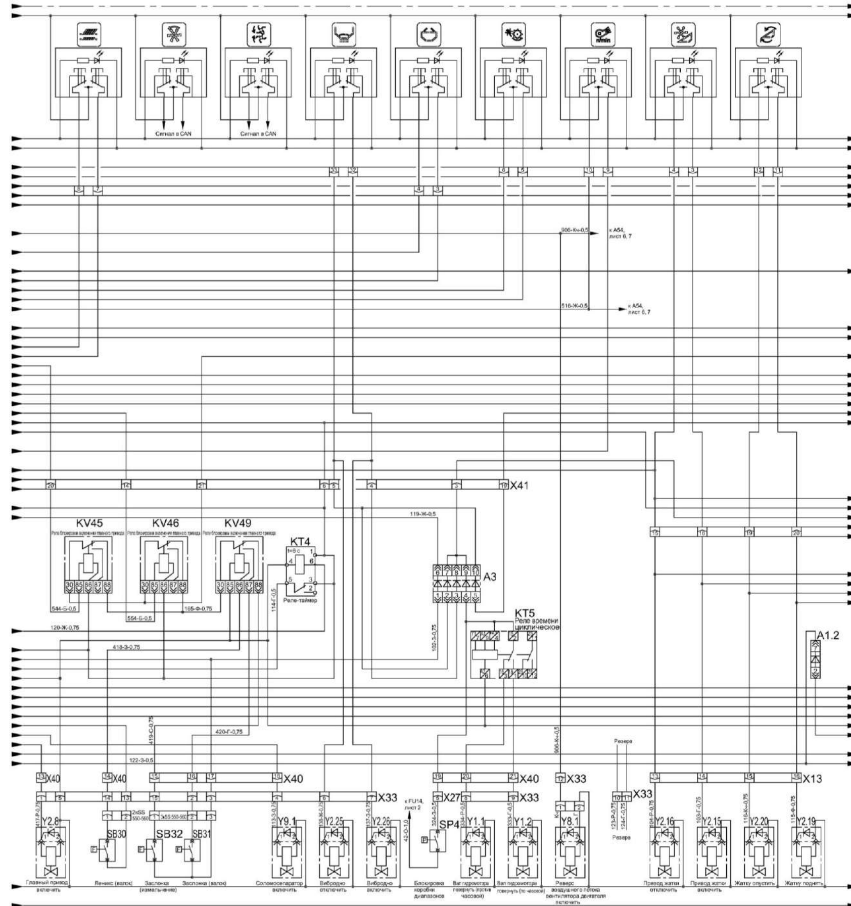
Рисунок Б.4 – Схема электрическая принципиальная комбайна (лист 3)
