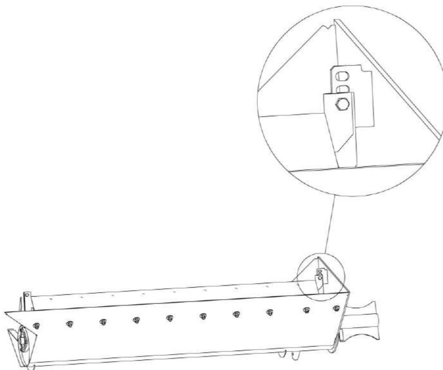
Рисунок 2.22 – Регулировка ограждения над горизонтальным шнеком бункера
