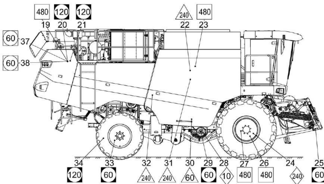
Рисунок 3.1 – Схема смазки комбайна (слева)
