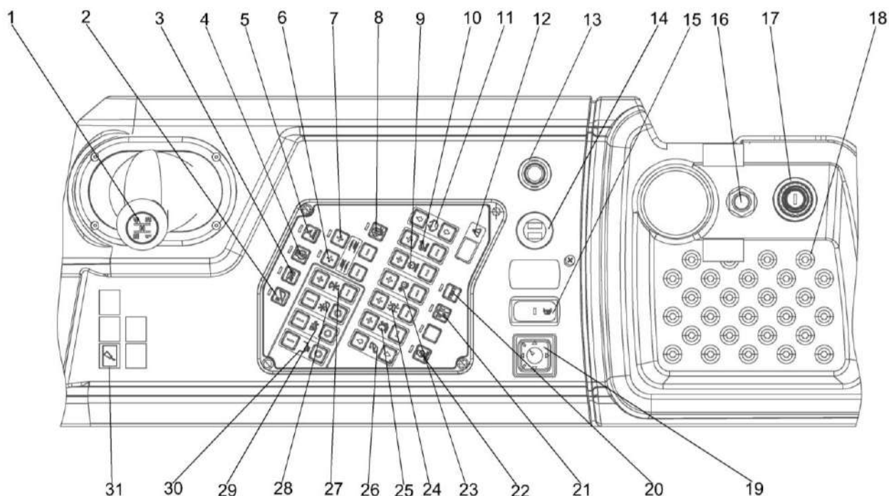
Рисунок 1.33 – Пульт управления комбайна
