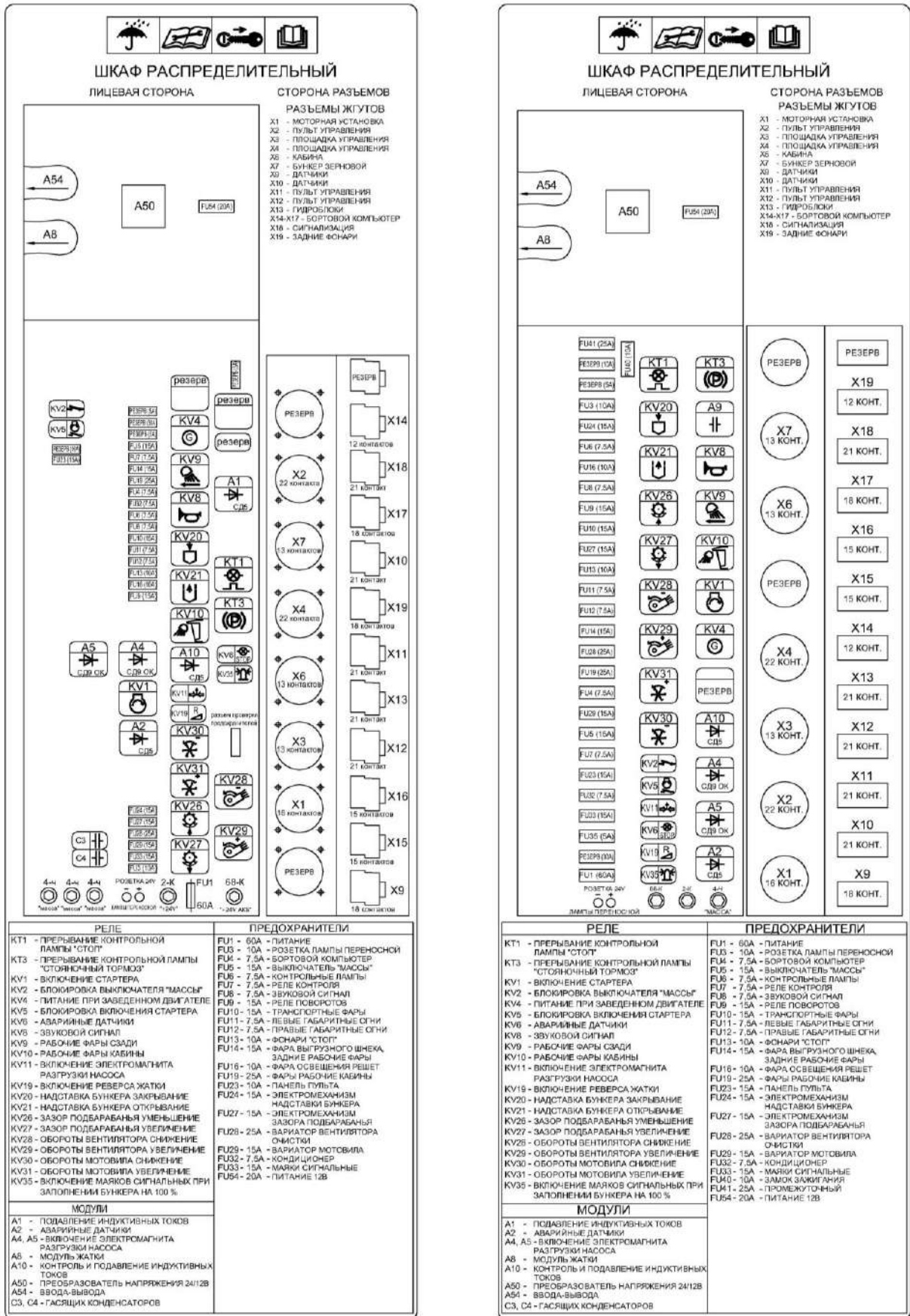
Рисунок 1.26 – Схема расположения элементов в электрошкафу
