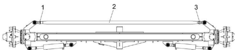
1, 3 – контргайки; 2 – рулевая тяга
