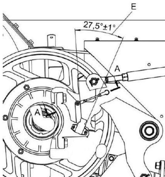
Расположение датчика В14
