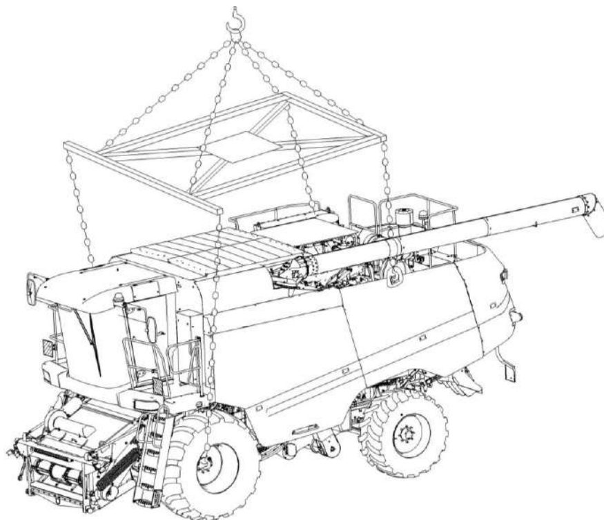
Рисунок 6.1 – Схема строповки комбайна
