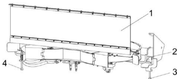
Рисунок 1.18 – Установка половоразбрасывателя
