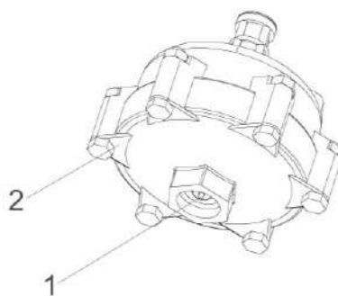
1 – шток; 2 – корпус
