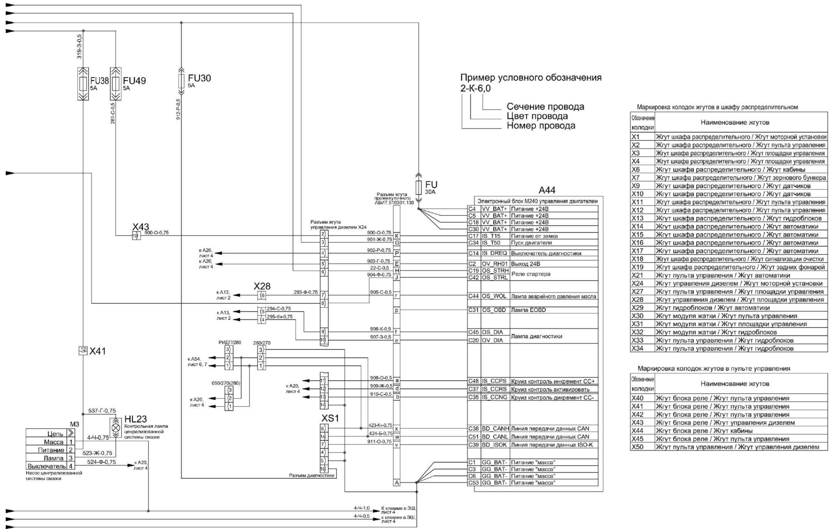
Рисунок Б.1 – Схема электрическая принципиальная комбайна (лист 2)
