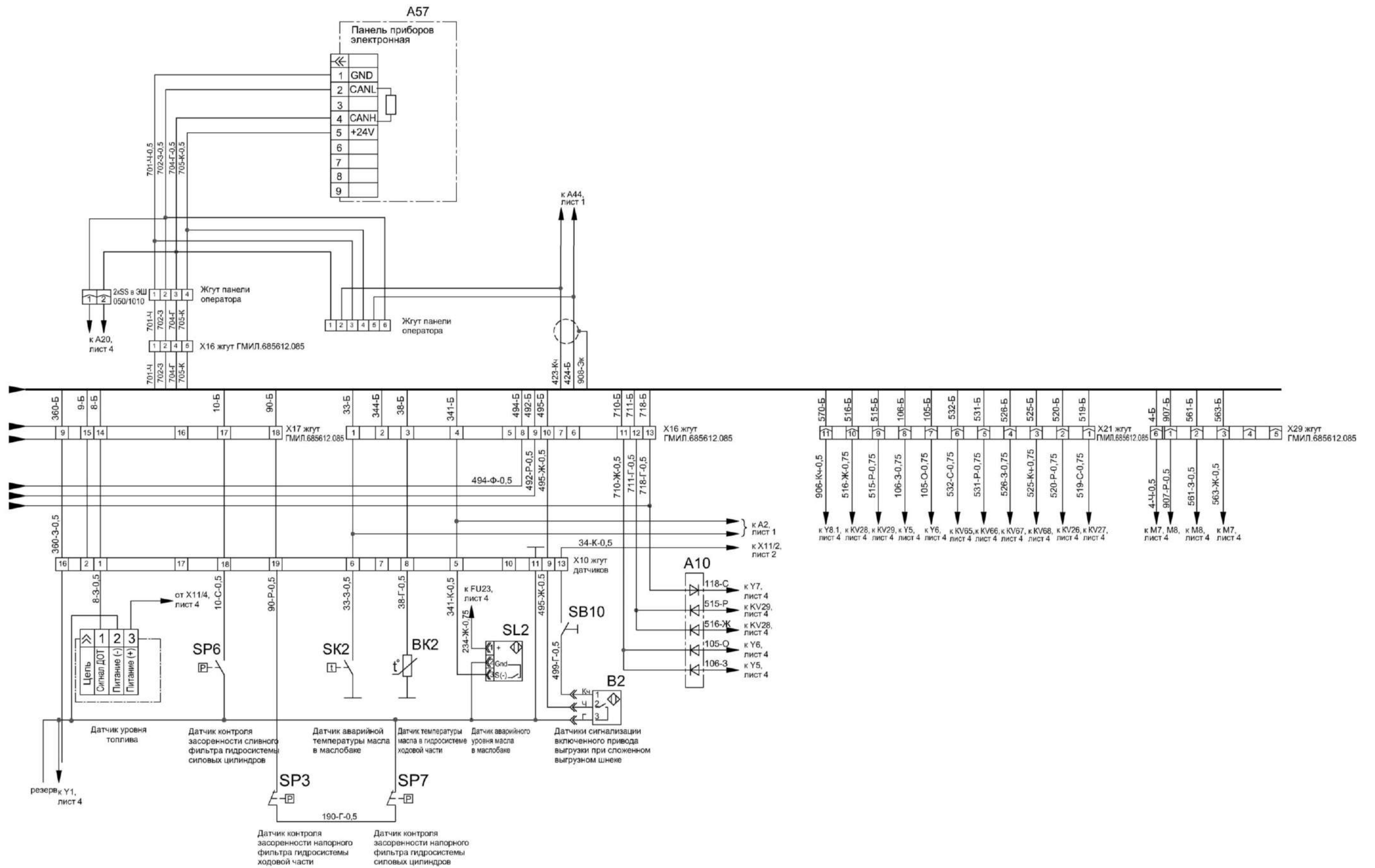
Рисунок Б.6 – Схема электрическая принципиальная комбайна (лист 2)
