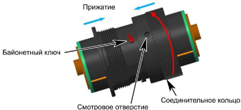
Рисунок 2.14 – Прижатие и проворот соединительного кольца
