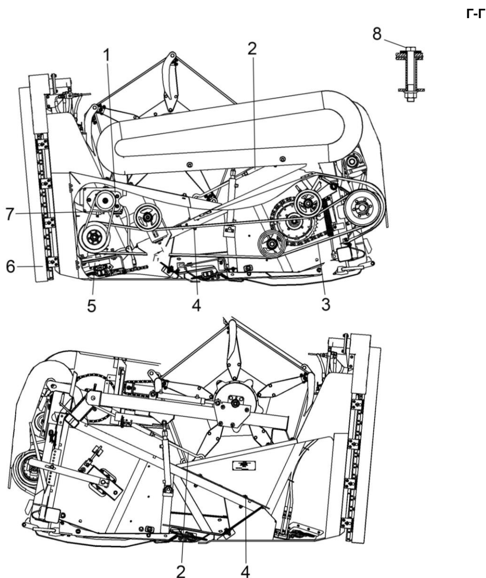
Рисунок 2.2 – Жатка для зерновых культур и приспособление для уборки рапса
