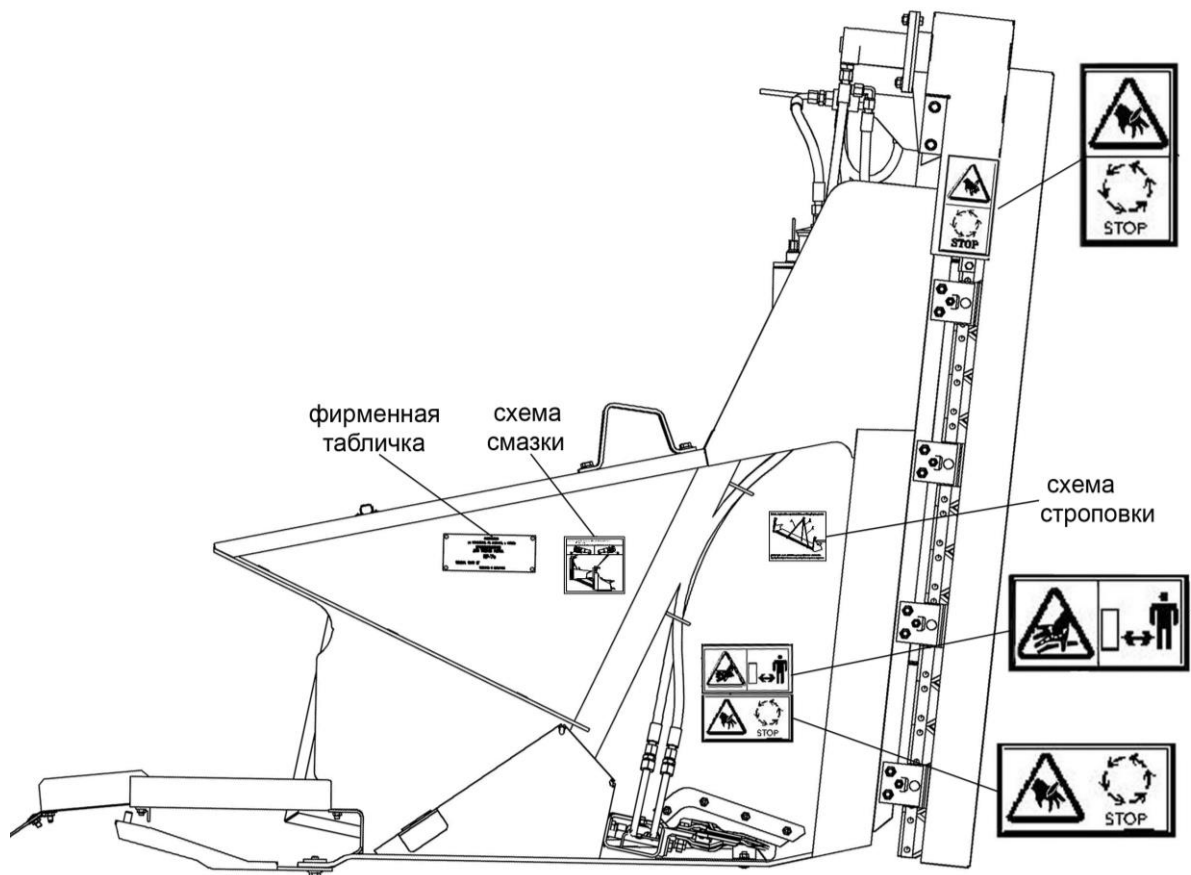
Расположение табличек на приспособлении (вид справа)
