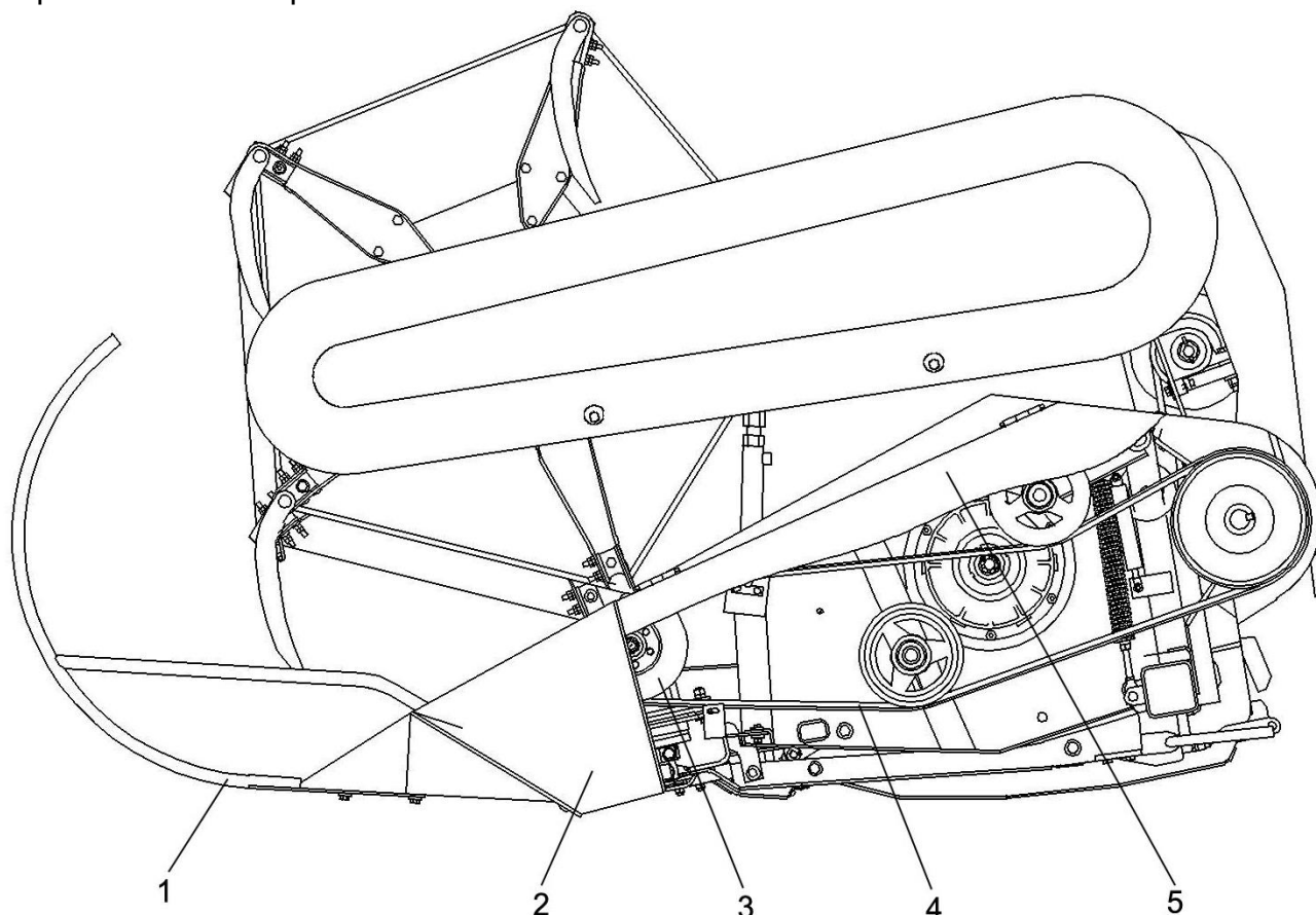
Рисунок 2.1 – Схема демонтажа жатки для зерновых культур
