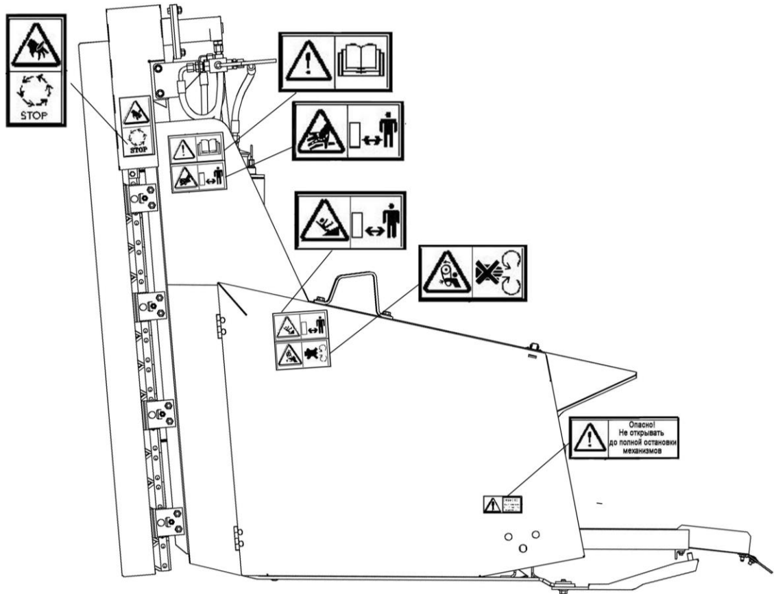
Расположение табличек на приспособлении (вид слева)
