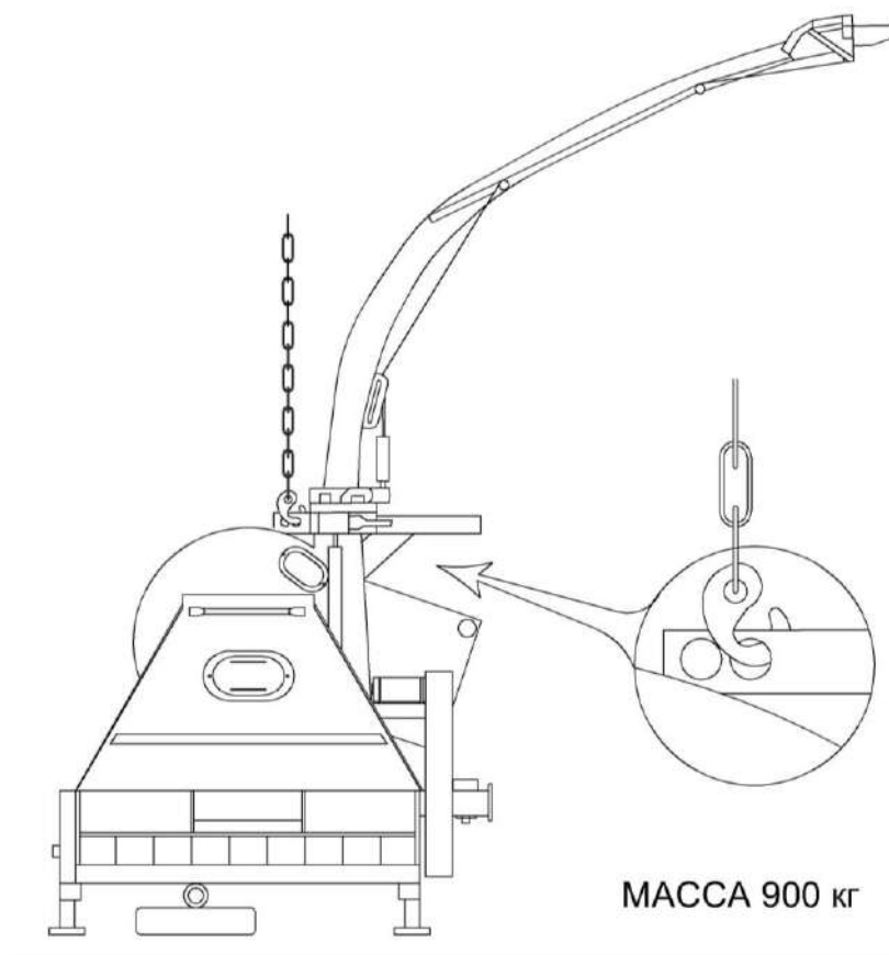
Рисунок 21 – Схема строповки
