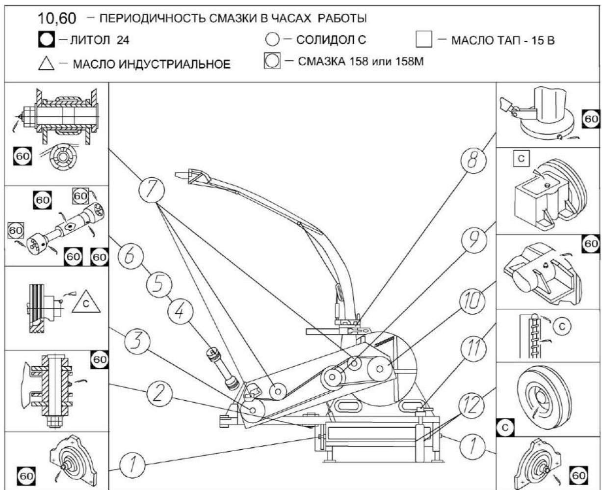
Рисунок 17 – Схема смазки
