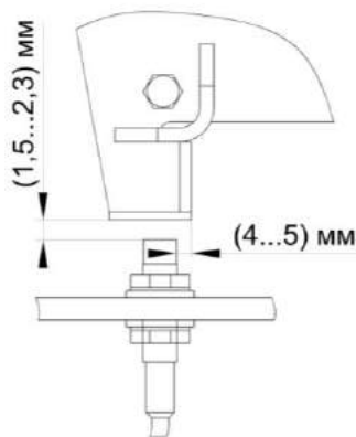
Рисунок 2.9– Установка датчика положения бруса абразивного
