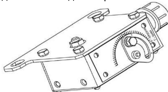
Рисунок 2.3 – Датчик камнедетектора
