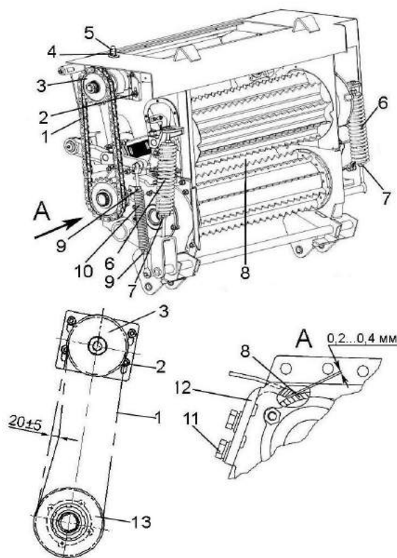
1 – цепь; 2, 4 – гайки; 3, 13 – звездочки; 5, 7, 9 – контргайки; 6, 10 – пружины; 8 – валец гладкий; 11 – болт; 12 – чистик Рисунок 2.11 – Аппарат питающий
