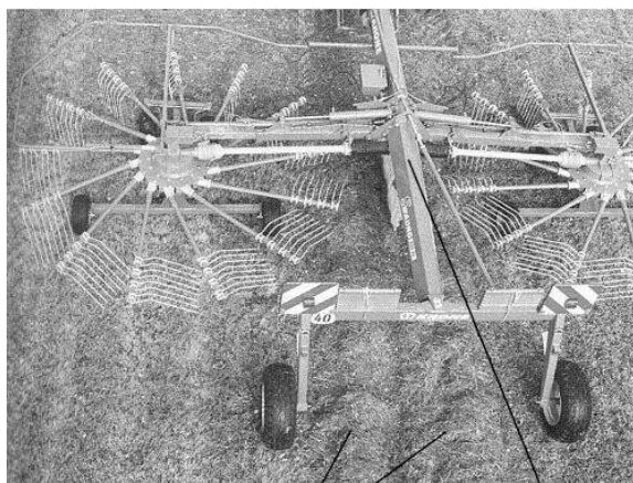
Рисунок 2.4 — Формирование валка при кослении
