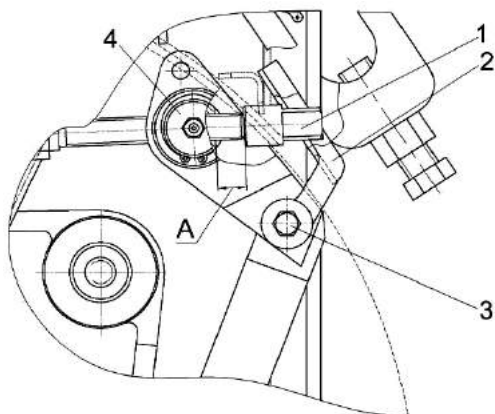
1 – втулка; 2 – скоба; 3 – болт; 4 – ось Рисунок 2.8 – Ручная регулировка зазора
