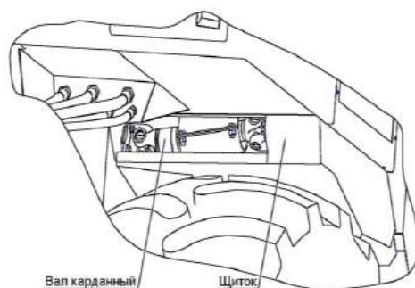
Рисунок 3.10 – Смазка шарниров карданного вала привода редуктора гидронасосов
