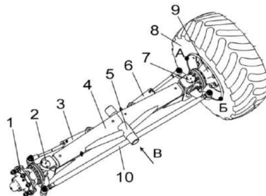
1, 9 – ступицы колес; 2, 7 – шкворни; 3, 6 – гидроцилиндры; 4 – балка моста; 5 – ось; 8 – колесо; 10 – тяга рулевая А и Б – условные отметки при регулировке сходимости колес;
