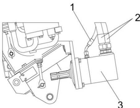
Рисунок 2.4 – Замена рукавов высокого давления
