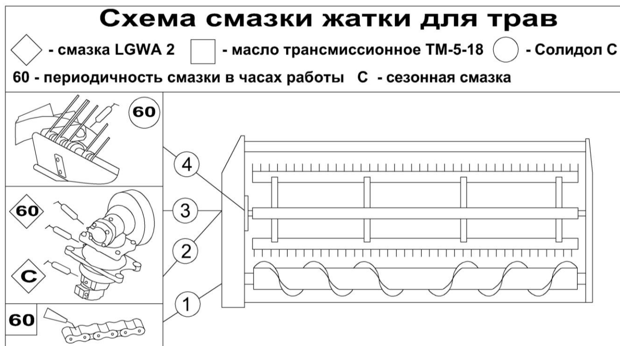
Рисунок 3.2 – Схема смазки жатки для трав
