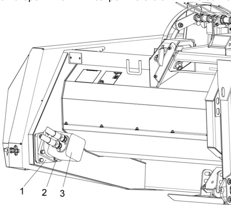
Рисунок 2.5 – Установка гидромотора привода жатки для трав
