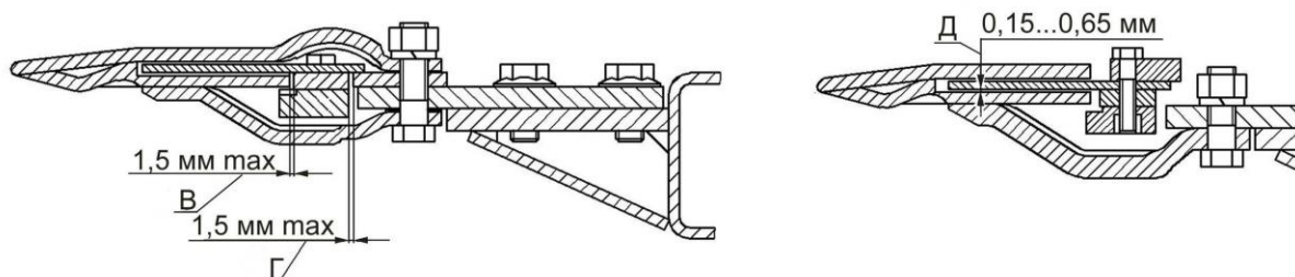
Рисунок 2.11 – Режущий аппарата
