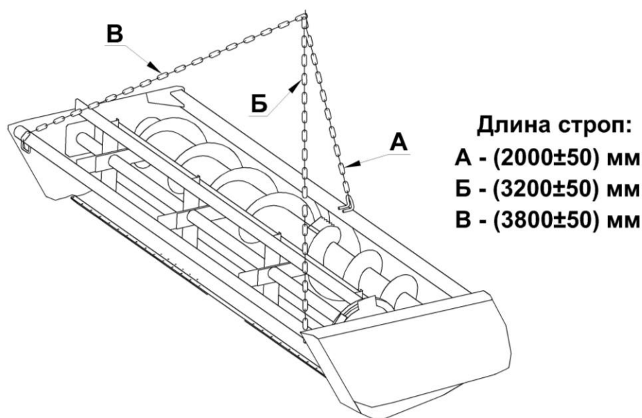
Рисунок 8.1 – Схема строповки
