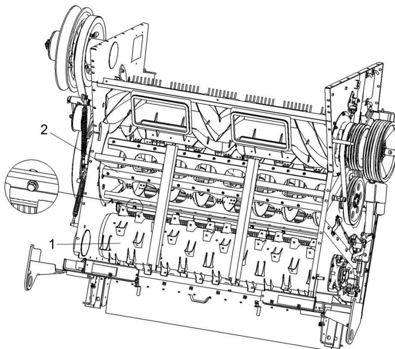
1 – барабан ускоряющий; 2 – барабан молотильный
