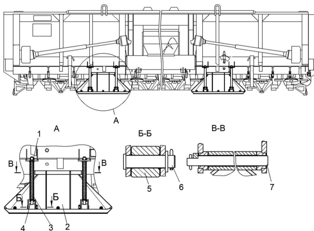
1 – втулка; 2 – лыжа; 3 – пружина; 4 – шайба; 5 – стойка; 6, 7 – оси
