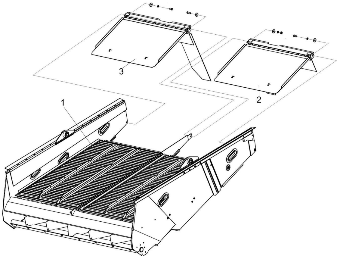
1 – решето нижнее; 2, 3 – заслонки половы
