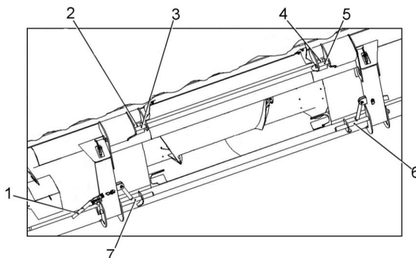
1 – рукоятка; 2, 4 – кулачки; 3, 5 – ловители жатки; 6, 7 – фиксаторы
