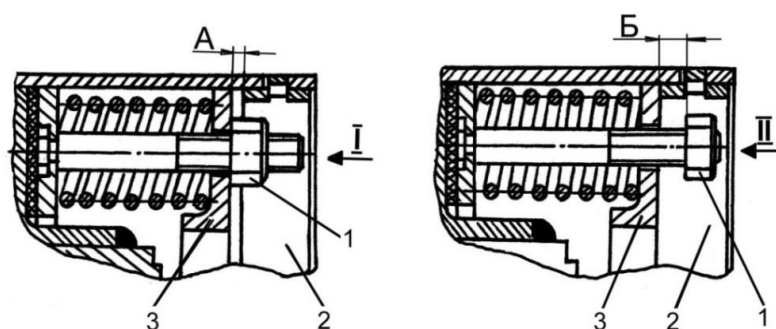
1 – гайка; 2 – замок; 3 – упорный диск
