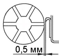
Рисунок 2.19 – Установка чистиков для очистки вальцов
