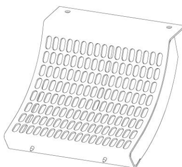
Рисунок 1.4 – Дека переднего подбарабанья
