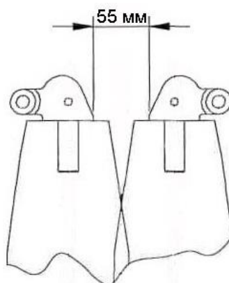
Рисунок 2.15 - Регулировка расстояния между корпусами подшипников вальцов
