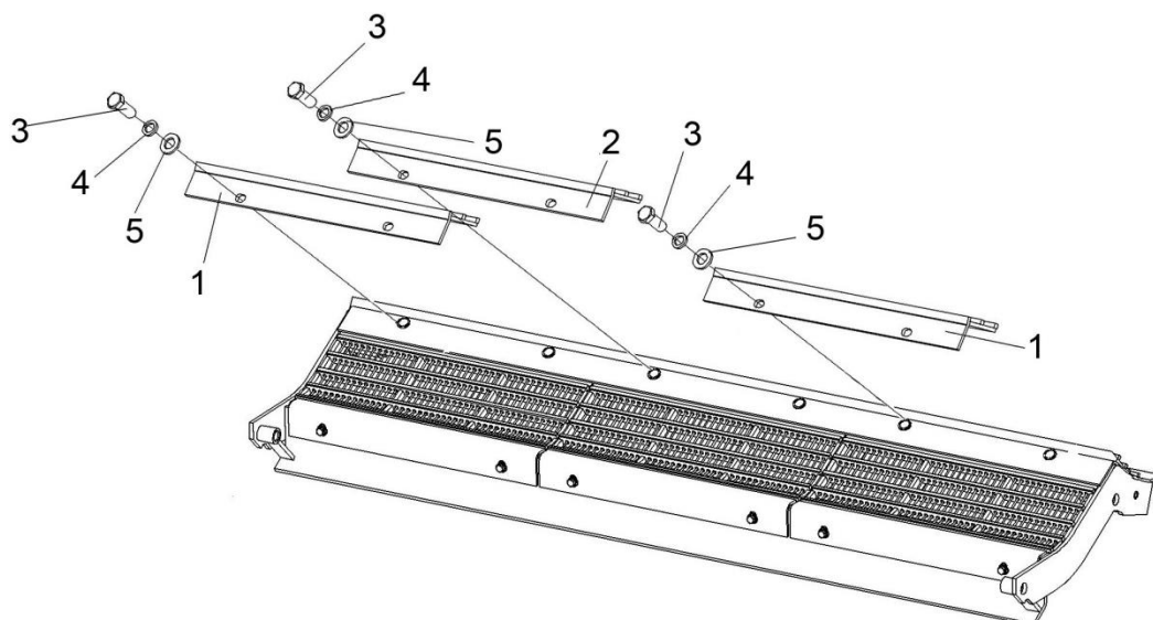
1, 2 – сегменты; 3 – болты; 4, 5 – шайбы
