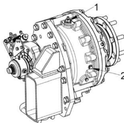
1 – отверстие для заправки; 2 – контрольное отверстие
