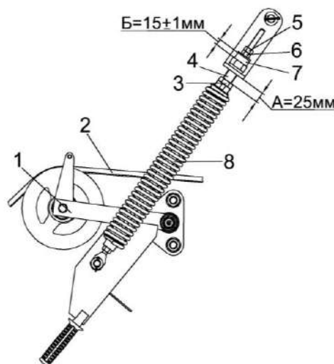
Рисунок 2.7 – Соломоизмельчитель
