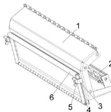
Рисунок 1.6– Аппарат молотильный
