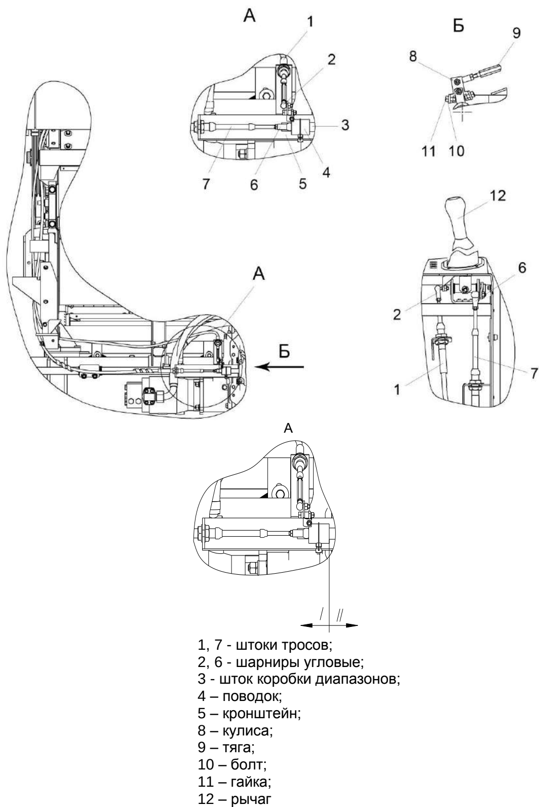
Рисунок 2.16 - Установка механизма переключения передач
