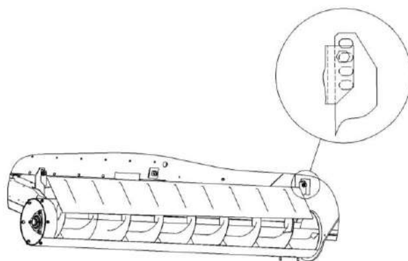
Рисунок 2.15 – Регулировка ограждения над горизонтальным шнеком бункера
