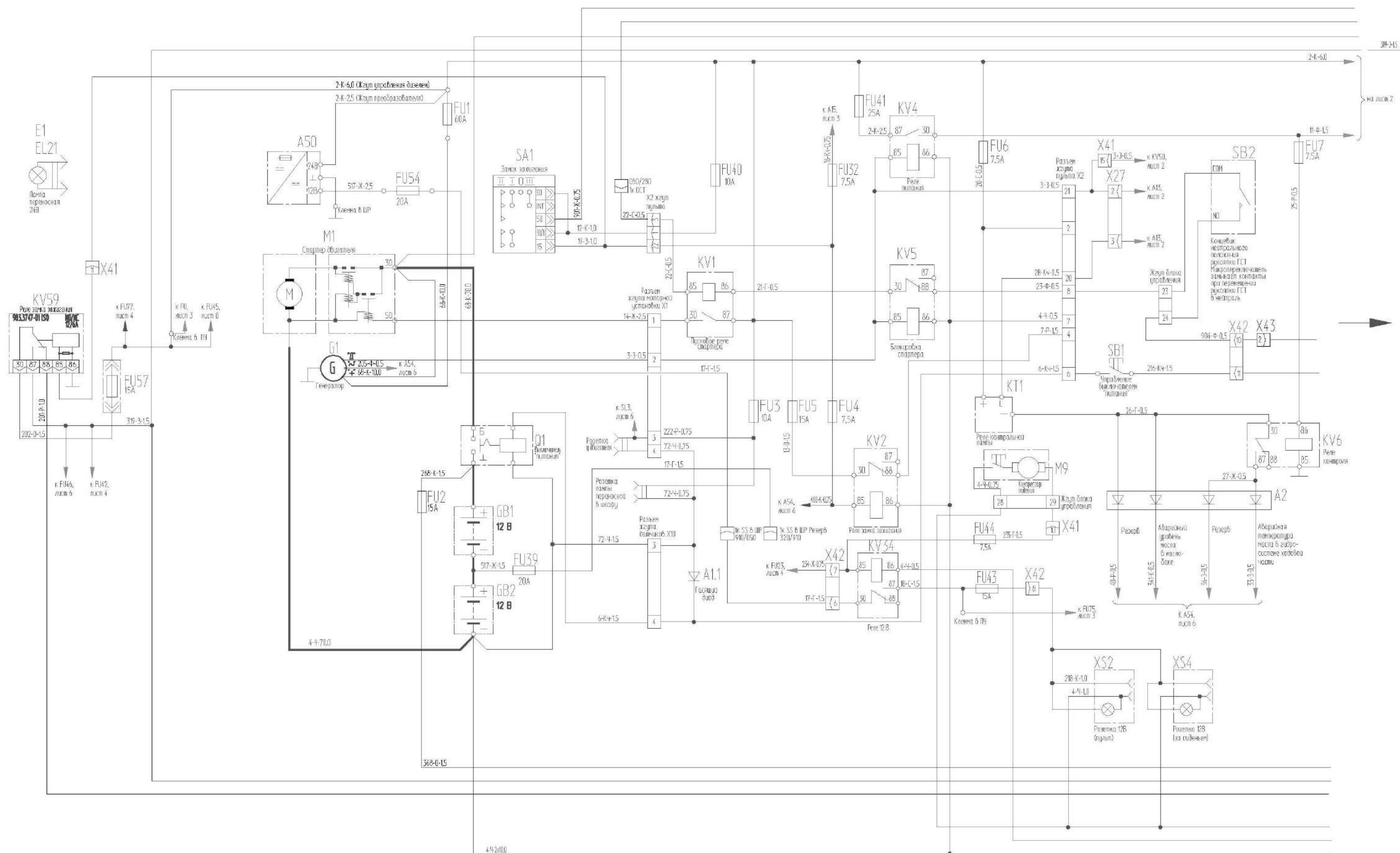
Рисунок Б.1 – Схема электрическая принципиальная комбайна (лист 1)
