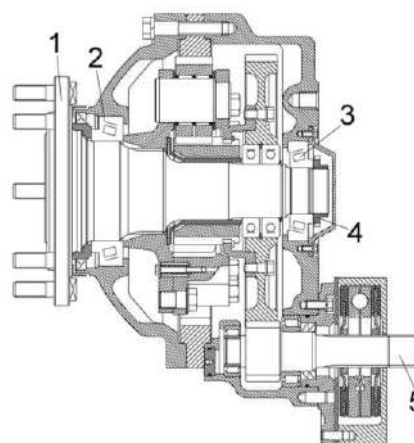
Рисунок 2.20 – Редуктор бортовой
