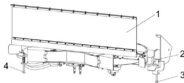
Рисунок 1.18 – Установка половоразбрасывателя
