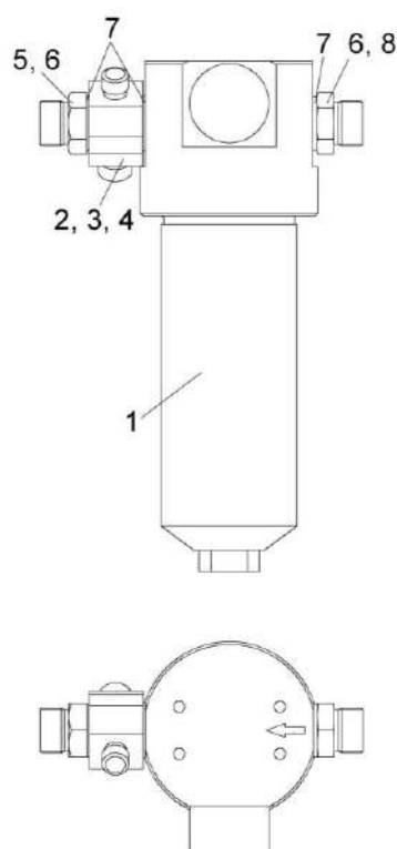
Рисунок 1.22 – Фильтр сливной
