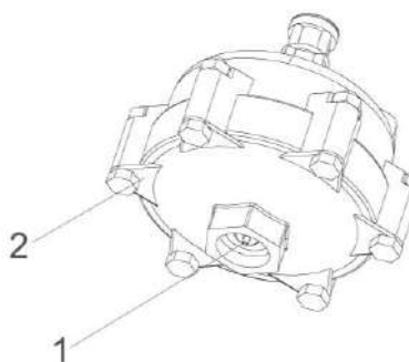
Рисунок 3.15 - Место установки клапана автоматического слива конденсата
