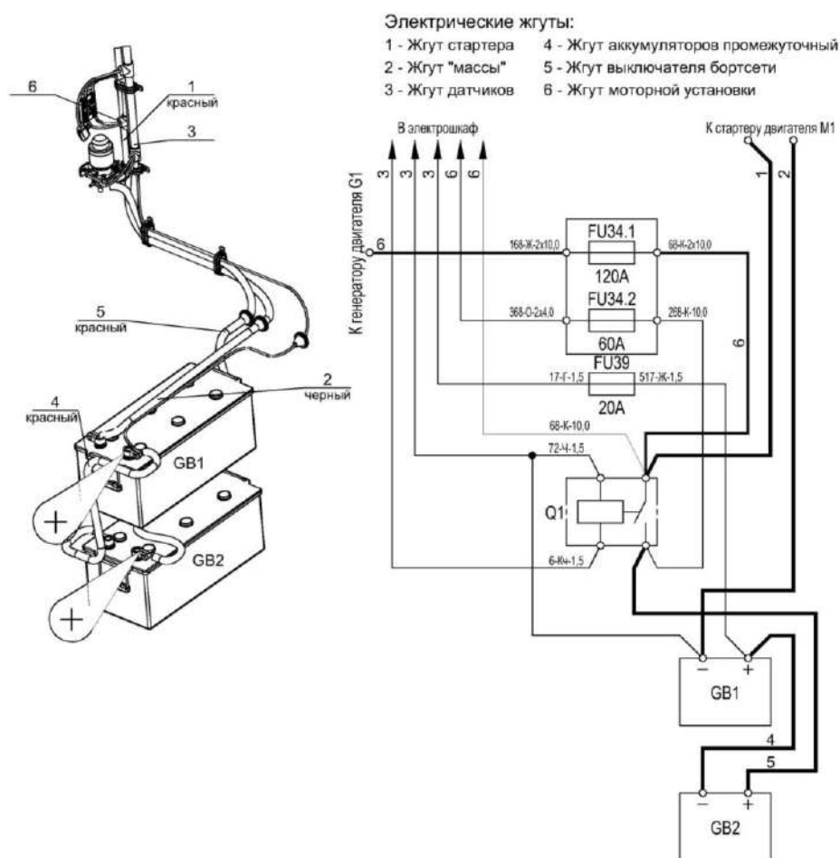
Рисунок 2.2 - Подключение аккумуляторных батарей
