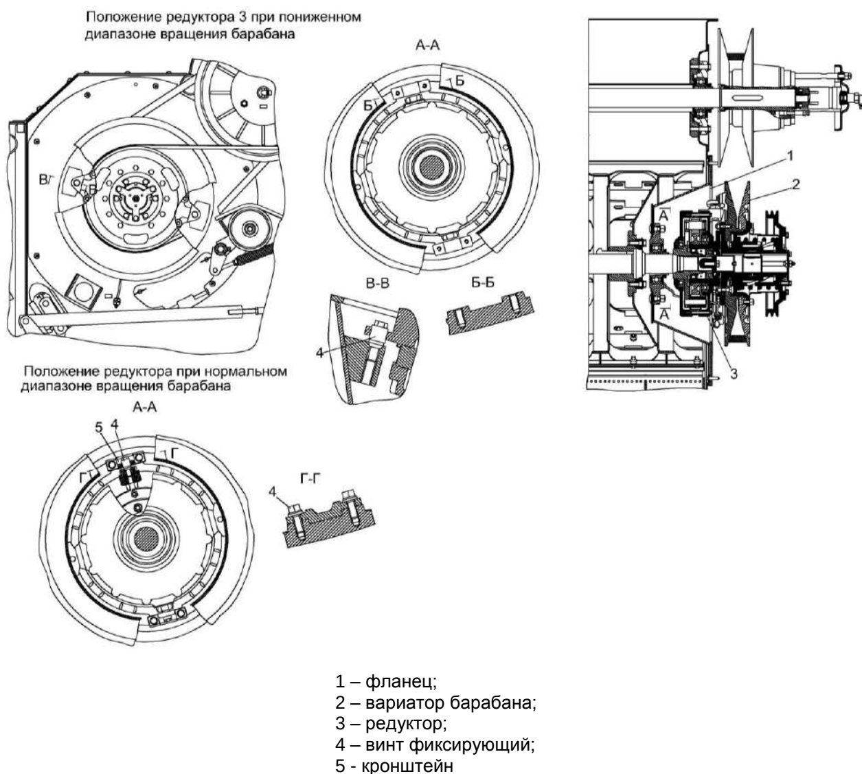
Рисунок 2.10 – Разблокировка понижающего редуктора
