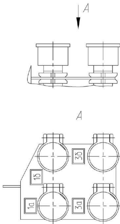
Рисунок 2.5 – Выводы гидросистемы косилки
