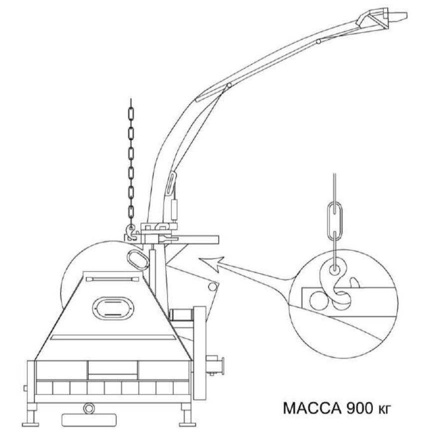
Рисунок 9.1 – Схема строповки
