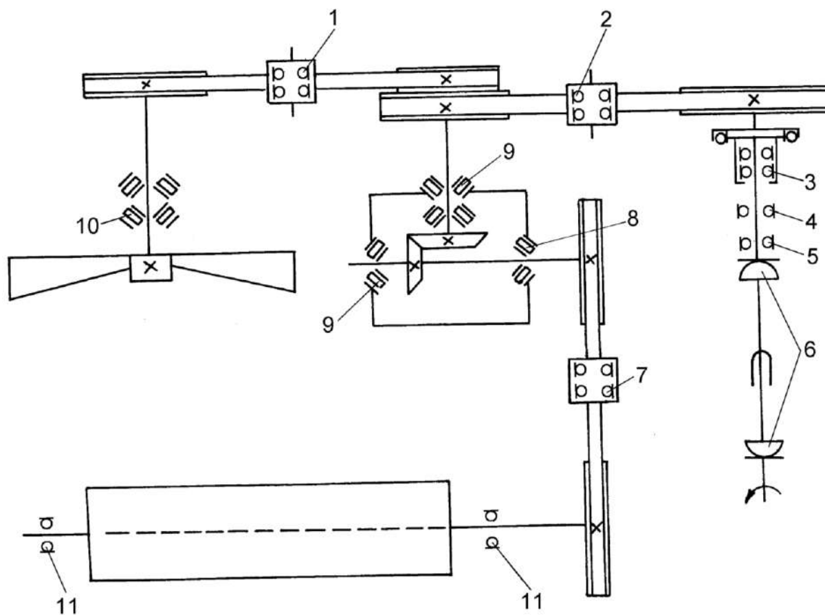
Рисунок Г.1 – Схема расположения подшипников
