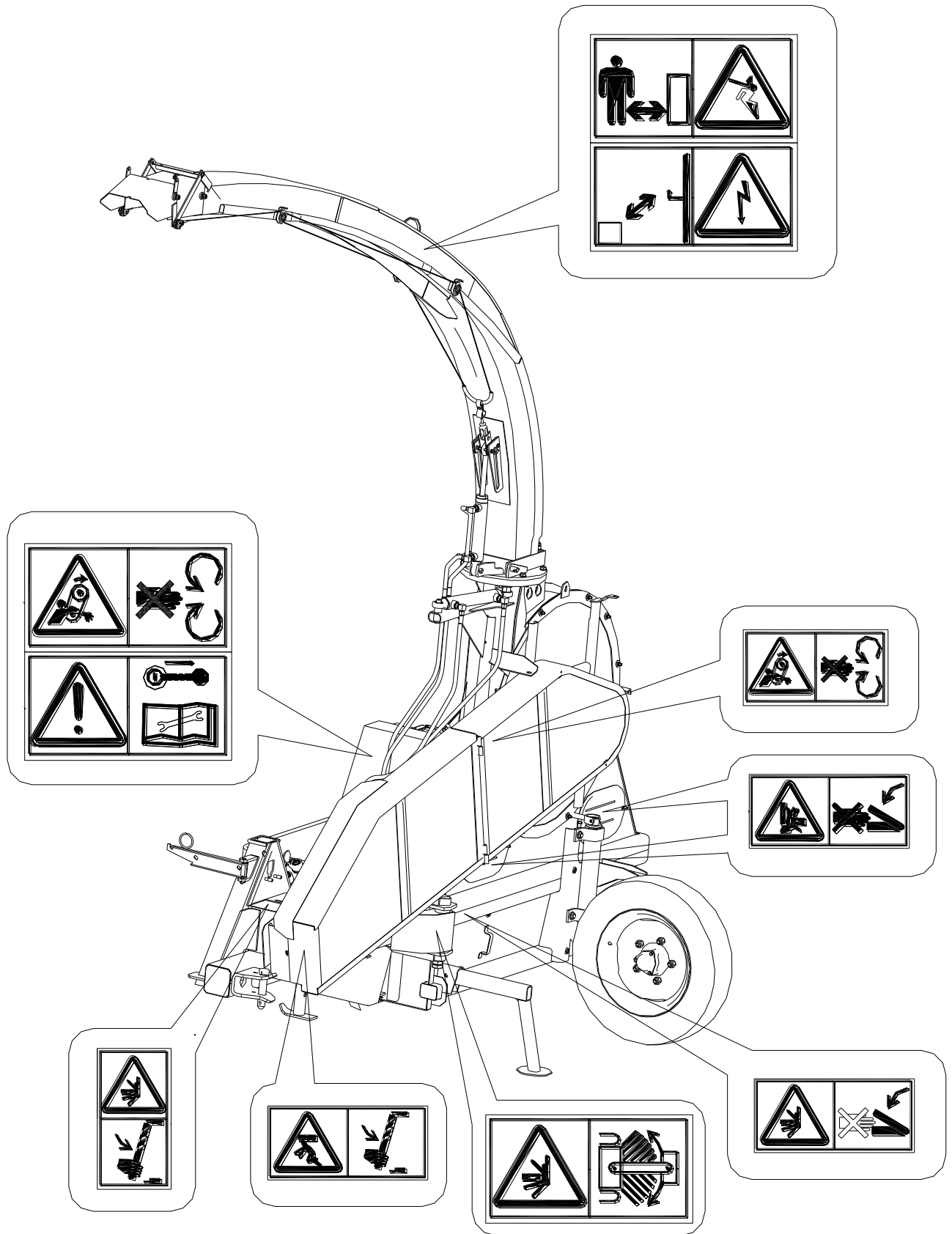
Знаки безопасности (пиктограммы) и их расположение на косилке
