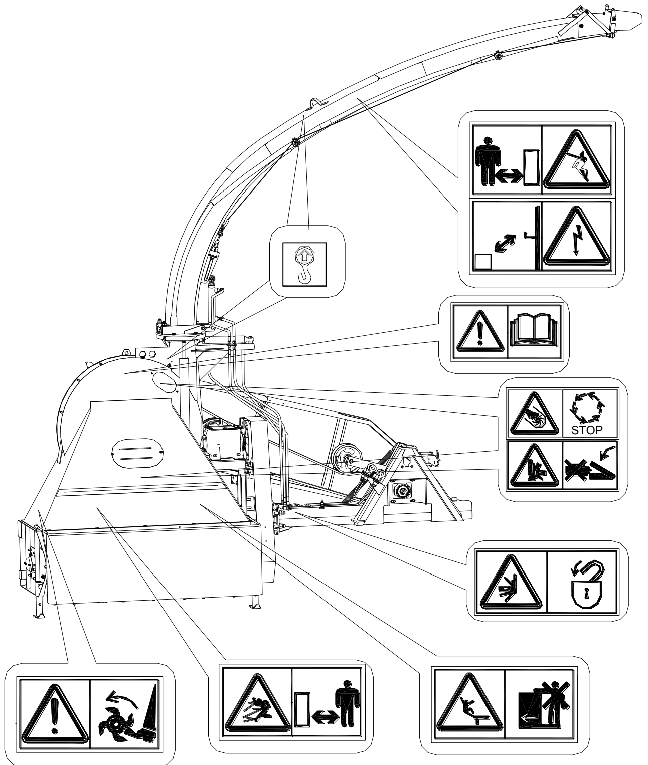
Знаки безопасности (пиктограммы) и их расположение на косилке
