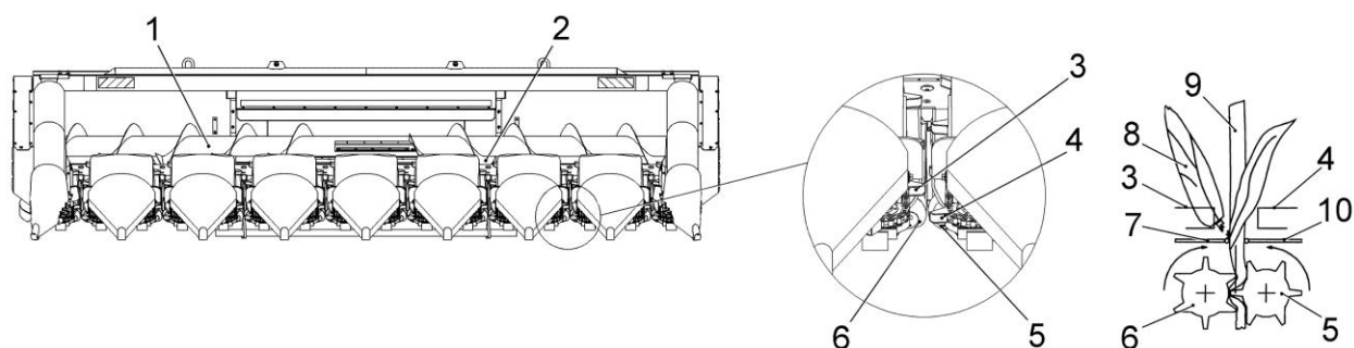
Рисунок 1.11 – Схема технологического процесса работы комбайна GS12A1 с комплектом
