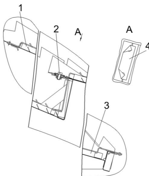
1, 3 – щиток, 2 – болт, 4 – пластина
