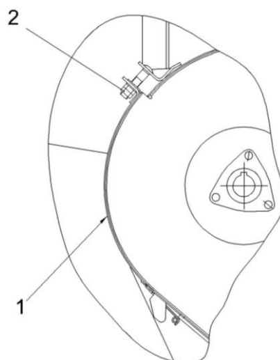
1 – крышка; 2 – гайка
