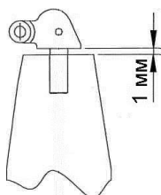
Рисунок 2.14 – Регулировка уплотнения типа «Лабиринт»
