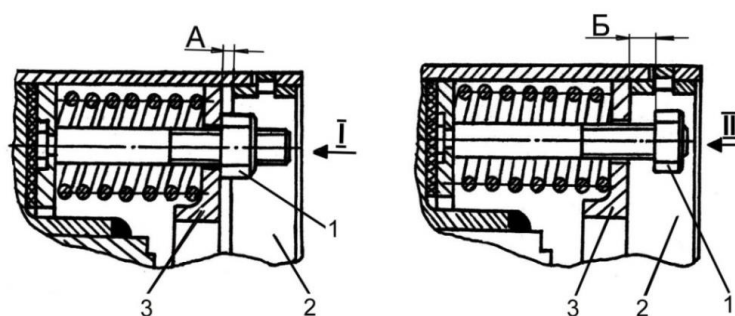
1 – гайка; 2 – замок; 3 – упорный диск
