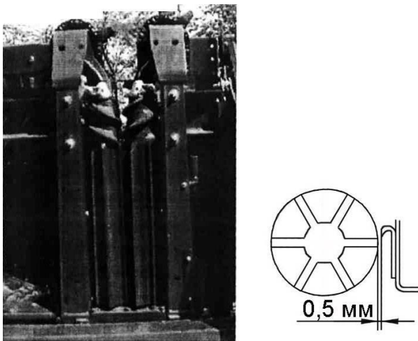
Рисунок 2.17 – Установка ножей для очистки вальцов
