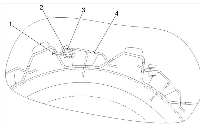
1 – планка упорная; 2 – болт; 3 – шайба; 4 – щиток перекрытия
