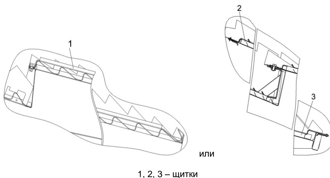
Рисунок 1.7 – Установка щитков перекрытия клавиш соломотряса
