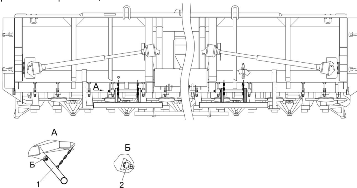
Рисунок 1.10 – Установка комплекта оборудования для загиба стерни КЗК 0805100
