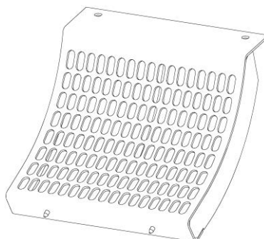
Рисунок 1.5 – Дека переднего подбарабья
