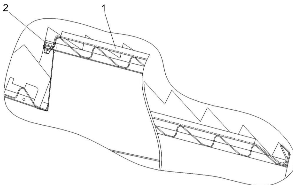
1 – щиток, 2 – болт
