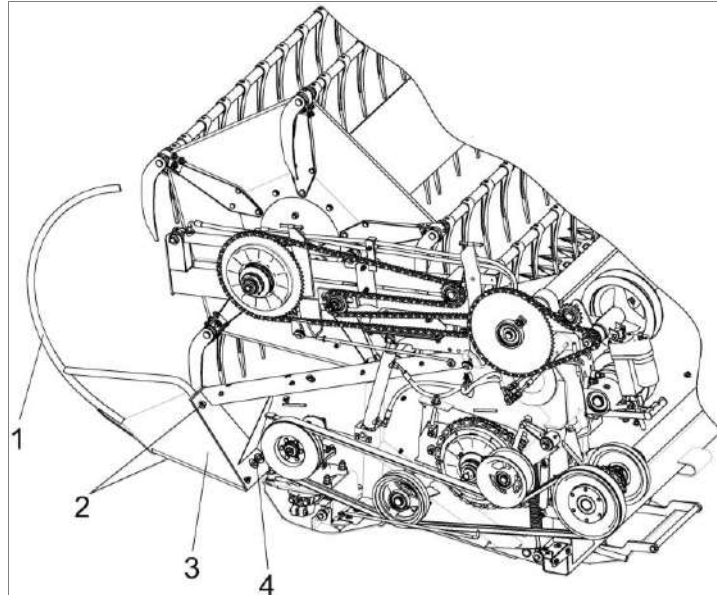
Рисунок 2.1 – Жатка
