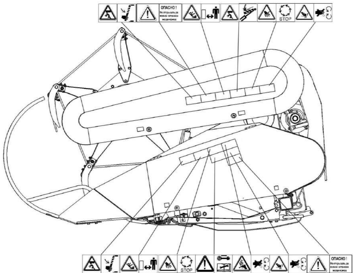
Жатка (вид слева)
